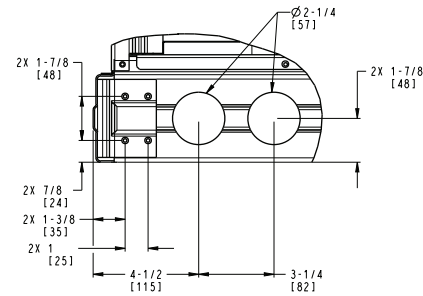
DETAIL A TYP 4 PLCS
