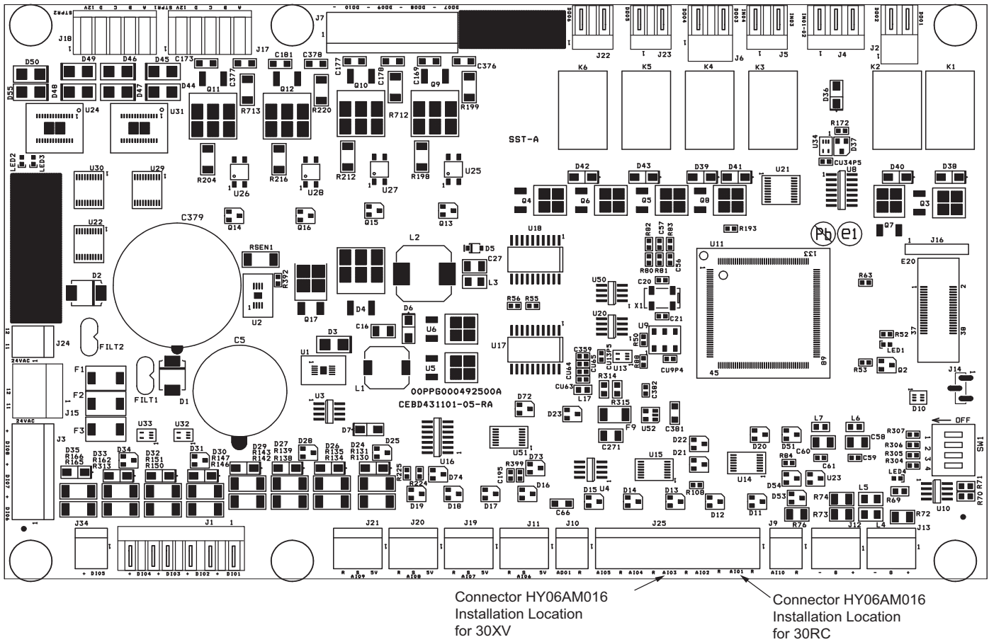
Fig. 5 — SIOB-B
