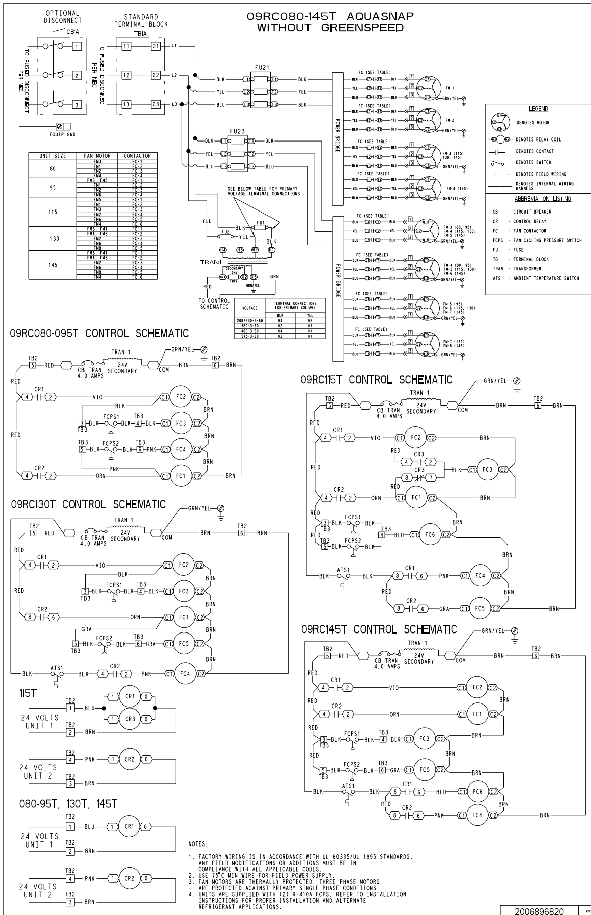
Fig. 36 — 09RC080-145 Fixed Speed Fan Control
