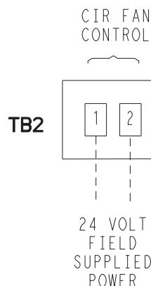
Fig. 28 — 09RC020-035 Control Circuit Wiring
