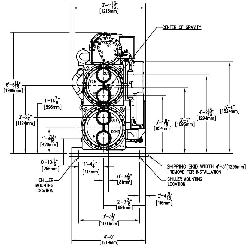
Fig. 5 — 30XW325-400 Unit Dimensions (cont)
