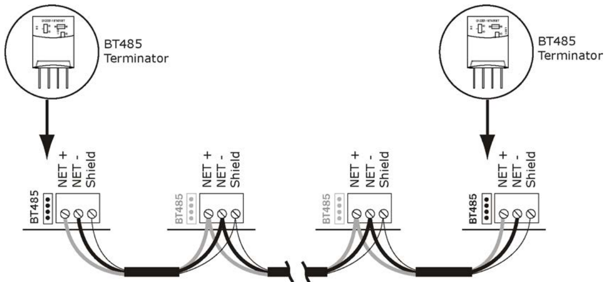
Fig. 23 —Network Wiring
