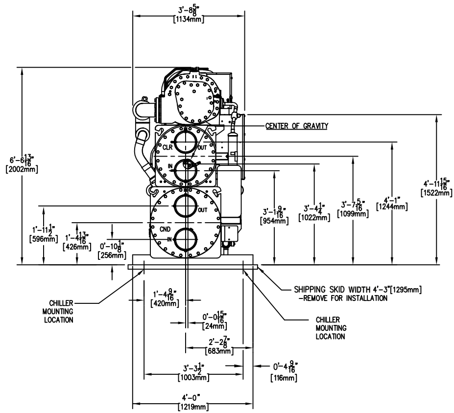
Fig. 4 — 30XW225-300 Unit Dimensions (cont)
