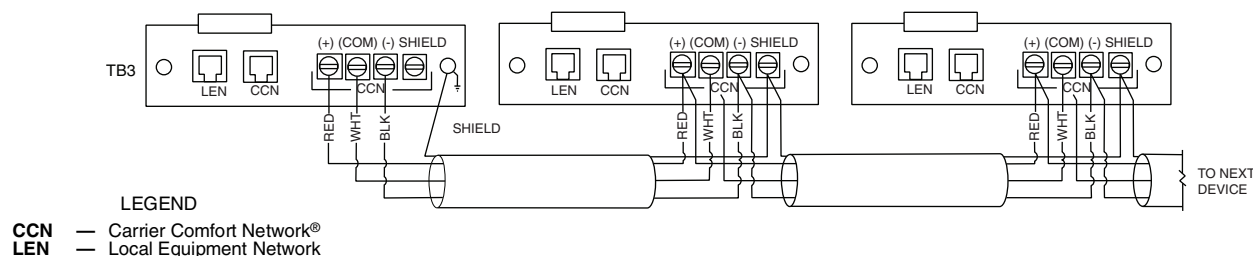
Fig. 21 — TB3 — CCN Wiring
