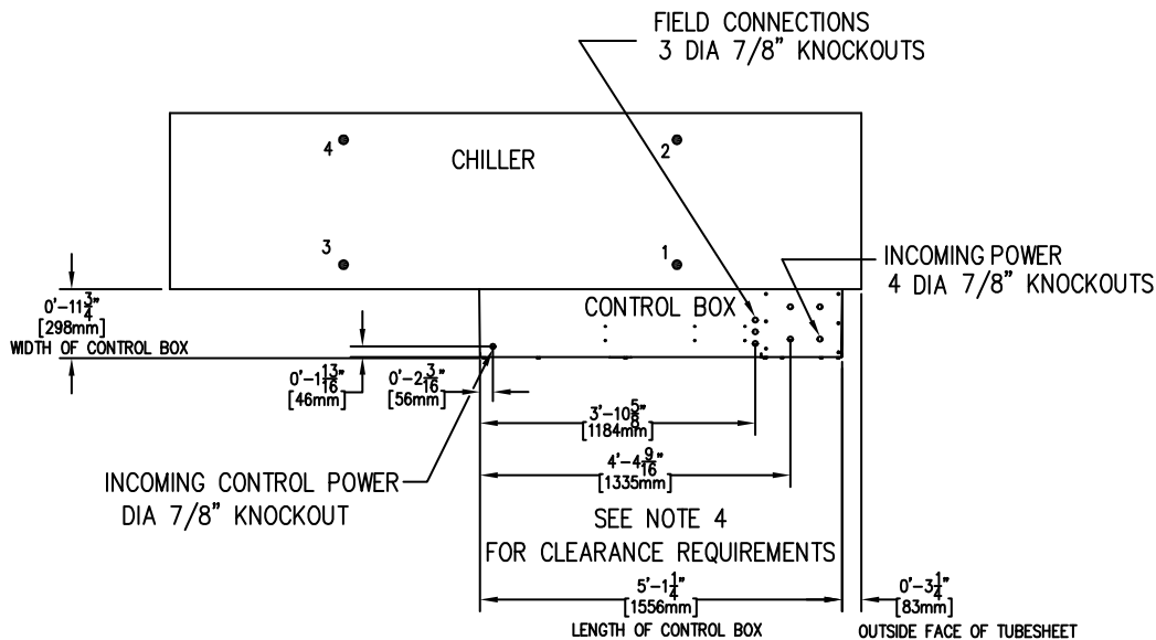
STANDARD 30XW150-200 UNIT DIMENSIONS
