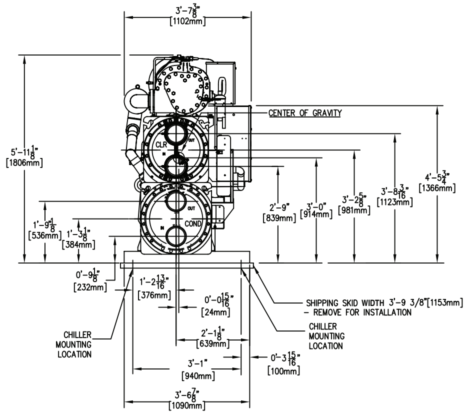
Fig. 3 — 30XW150-200 Unit Dimensions (cont)
