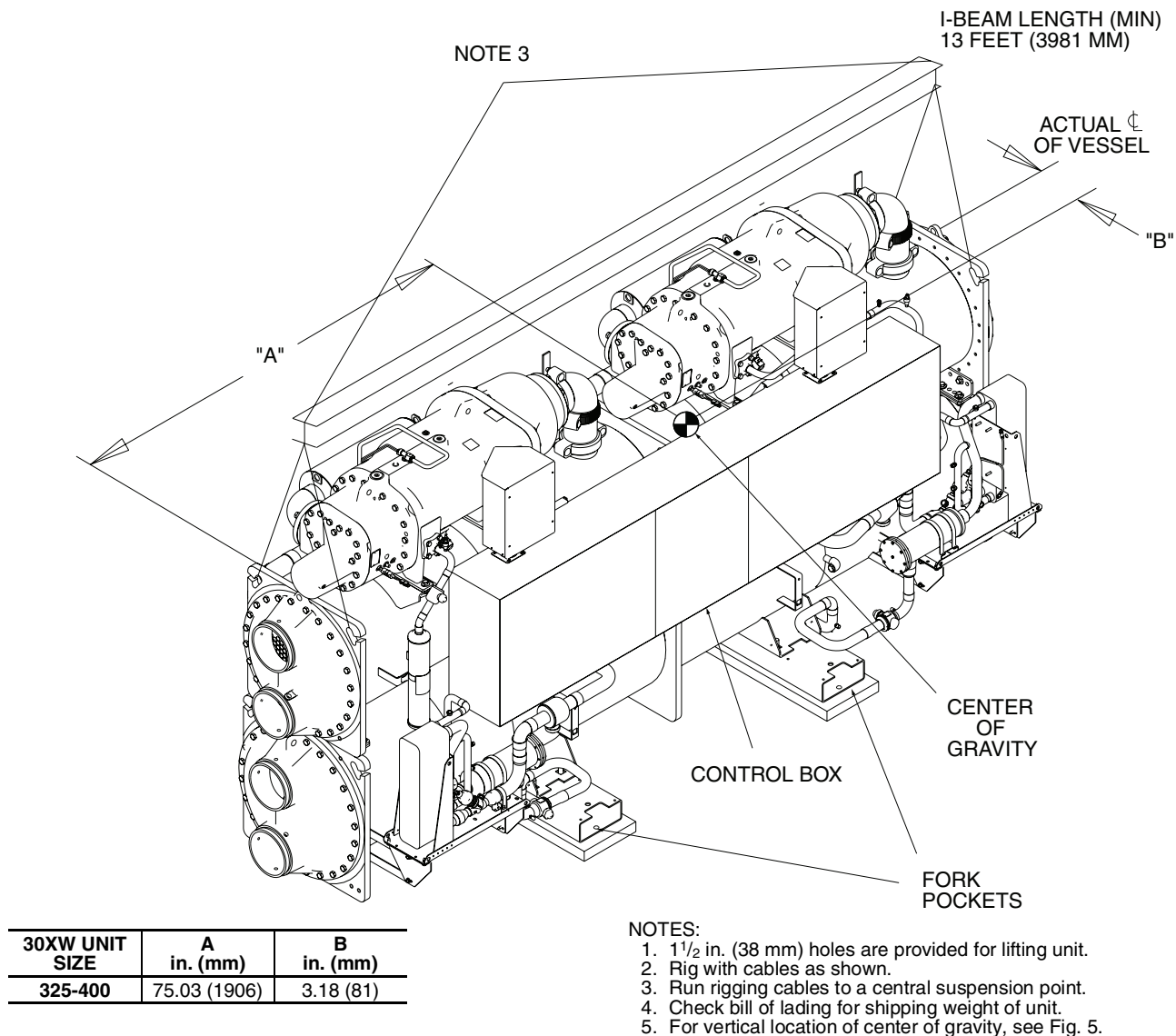
Fig. 9 — 30XW325-400 Unit Rigging
