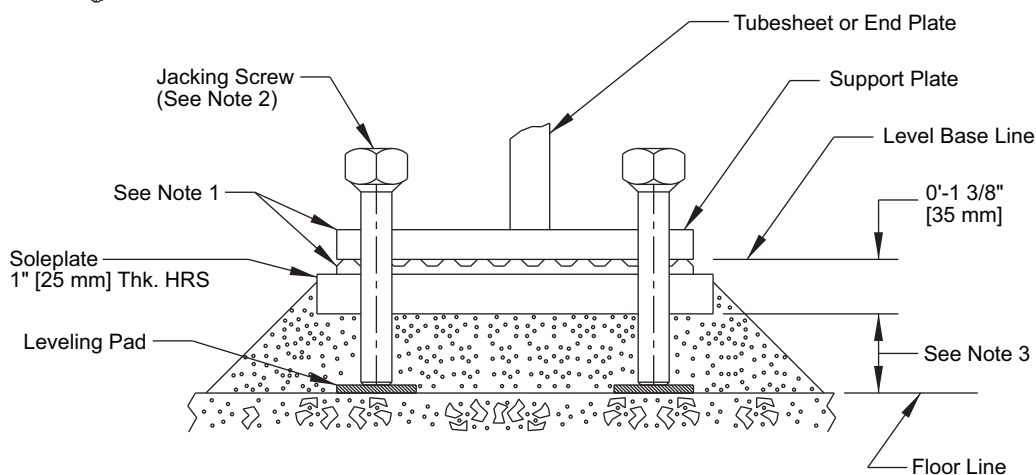
VIEW A-A
