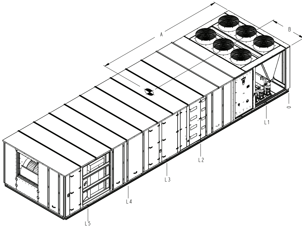
Fig. 7 — 48N 75-150 Ton Non-Split Rigging
