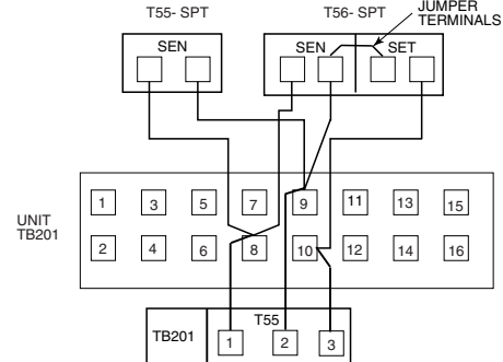
Fig. 48 — T-55 or T-56 Wiring
