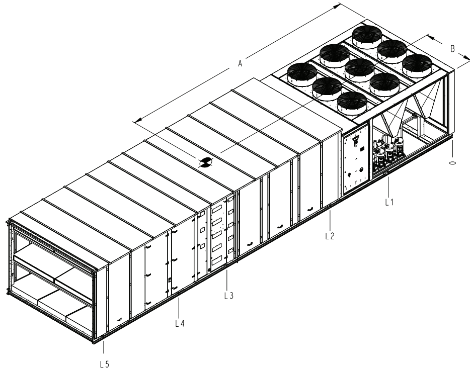
Fig. 8 — 48N 75-150 Ton Split (Main Unit) Rigging
