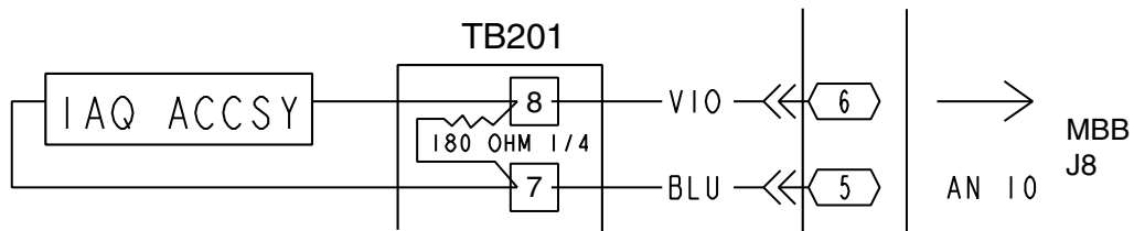
Fig. 52 — CO 2 Space Sensor Wiring
