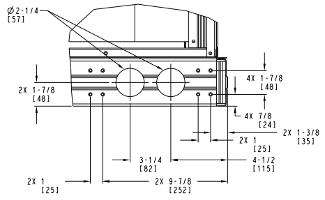
DETAIL A TYP 4 PLCS
