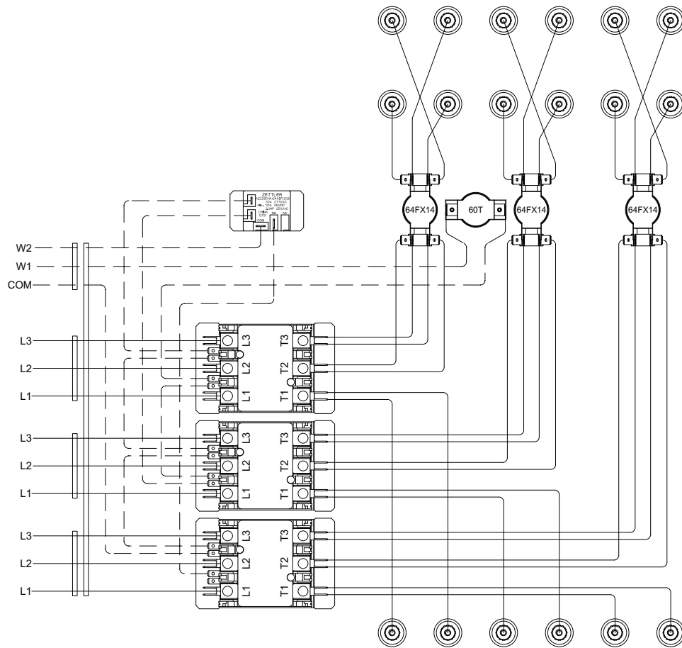
Fig. V — CRHEATER416A, 417A, 452A, 453A Wiring Assembly
