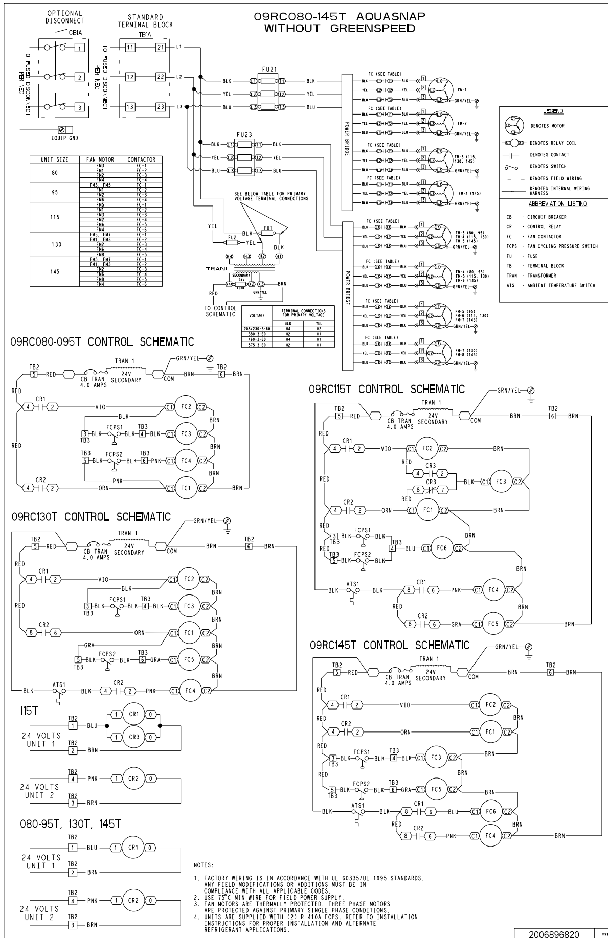
Fig. 38 — 09RC080-145 Fixed Speed Fan Control
