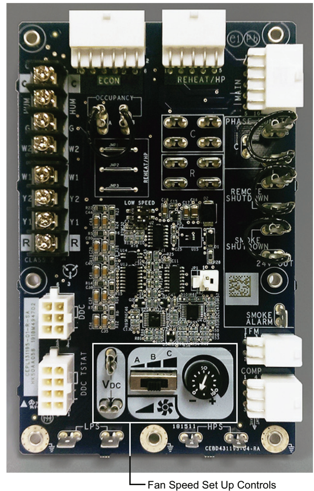
Fig. 23 — UCB Fan Speed Controls
