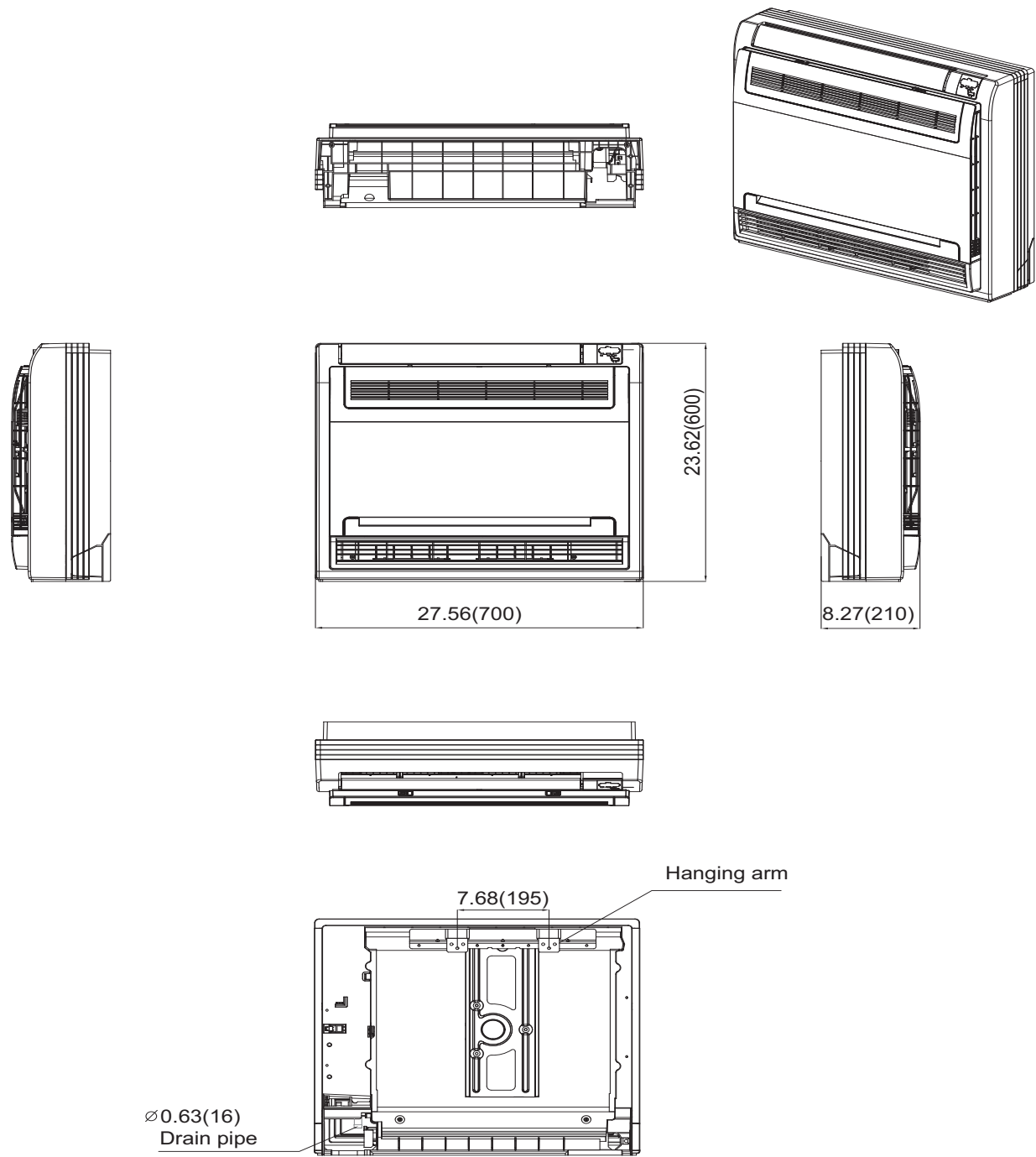
Fig. 2 – Indoor Unit
