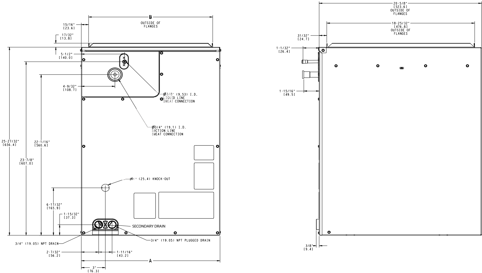
Fig. 10 – CSPVA
