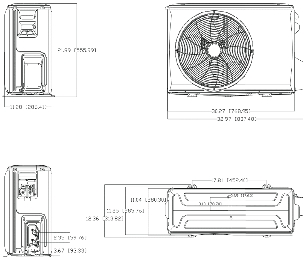
Fig. 2 – Size 6K / 9K / 12K
