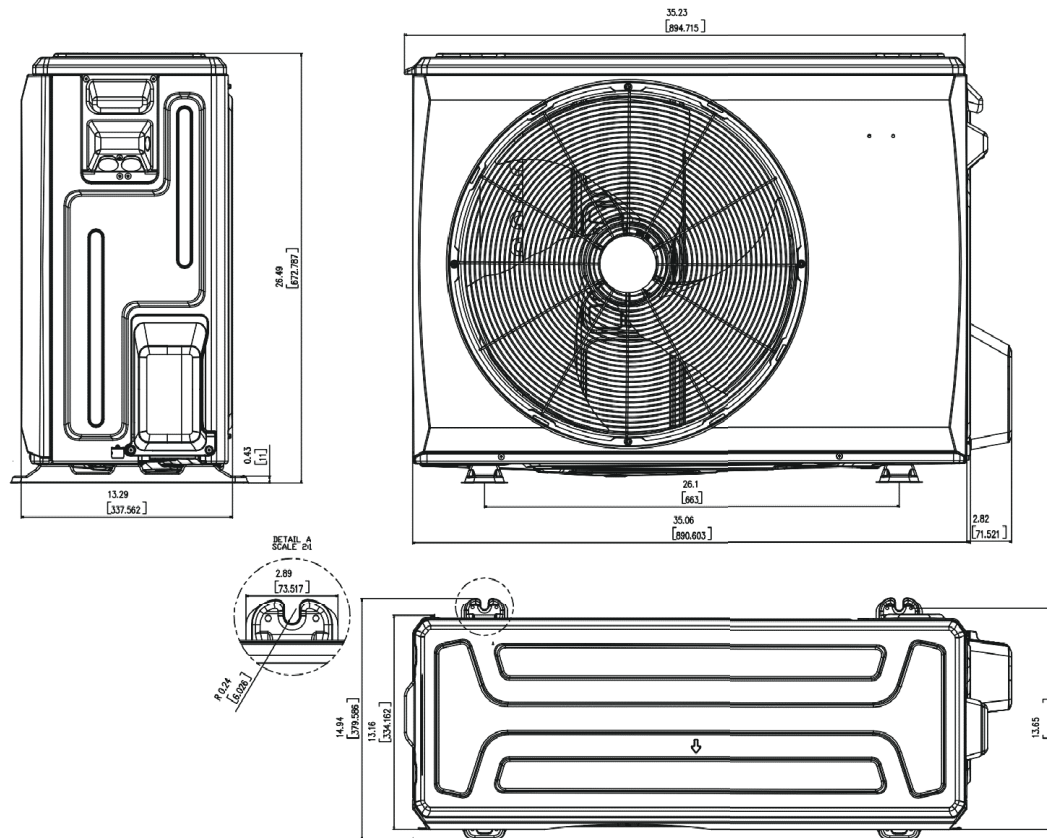
Fig. 3 – Size 18K
