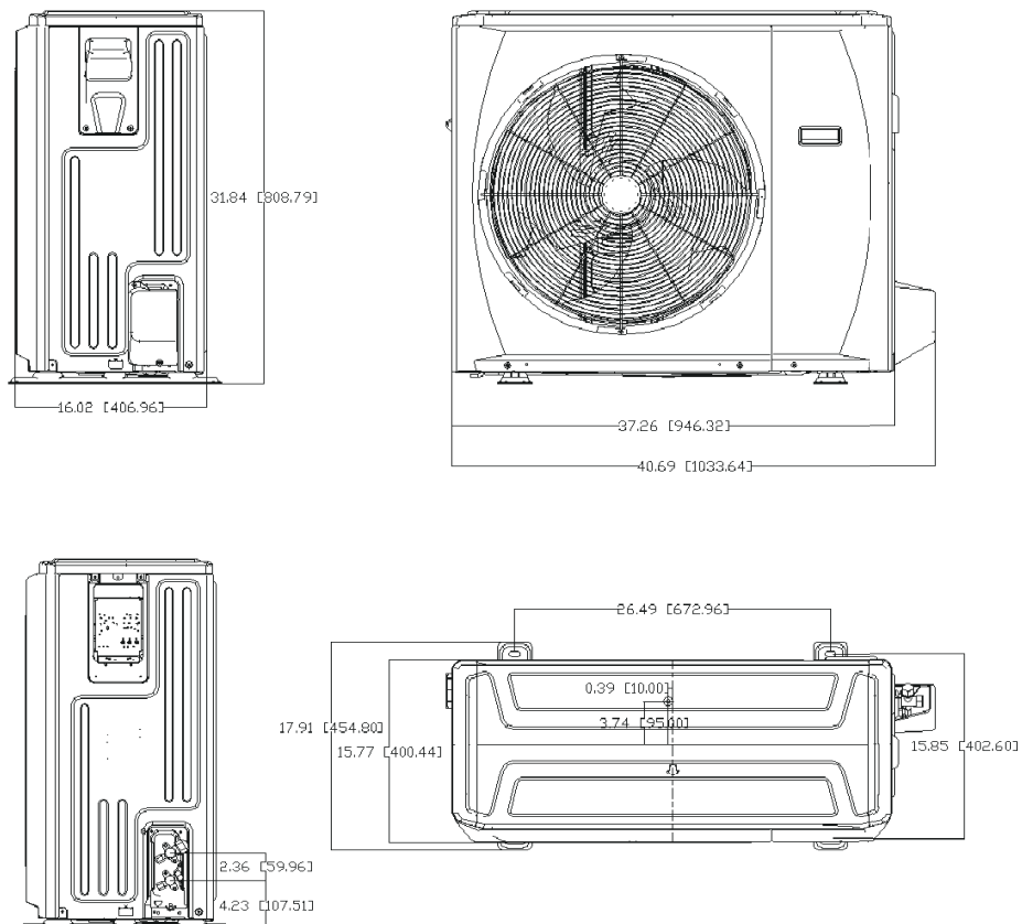
Fig. 3 – Size 18K
