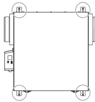
INSTALLATION AVEC 4 SUPPORTS
