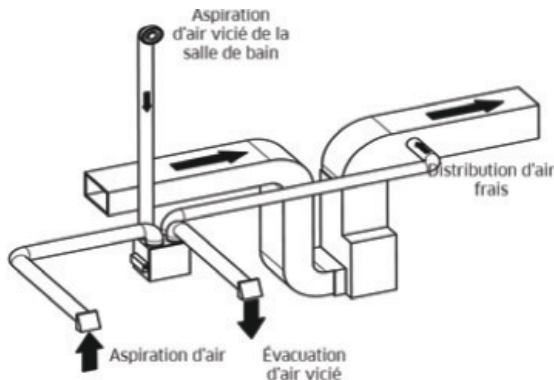
Fig. 7 – Système d'Évacuation – Alternative
