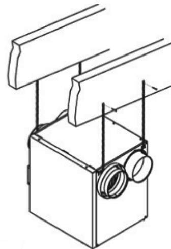
Fig. 2 – Choisir un Emplacement Adéquat pour l'Appareil Installé au Mur:
