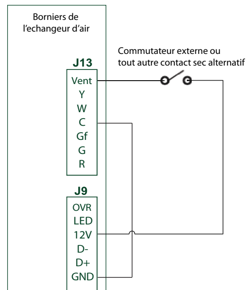
Fig. 17 – Câblage Pour Connexion Par Contact Sec
