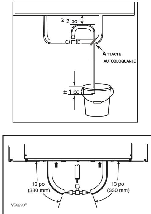
Fig. 10 – Connexion de Vidange
