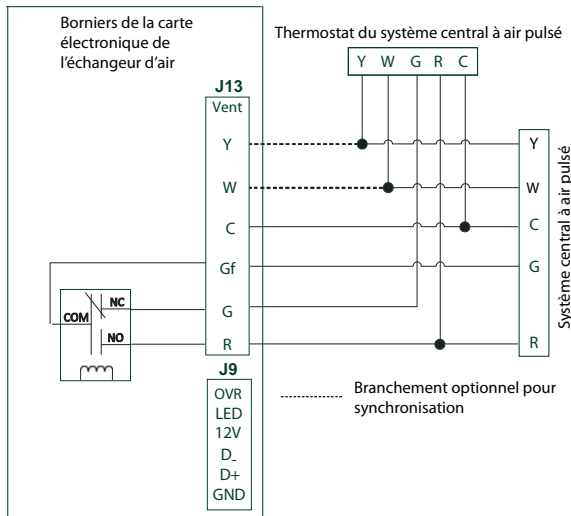
Fig. 19 – Options de Câblage Avec Système Central à Air Pulsé
