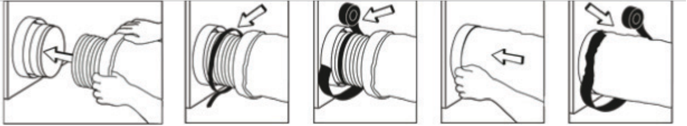
Fig. 13 – Connectez le Conduit à l'Unité
