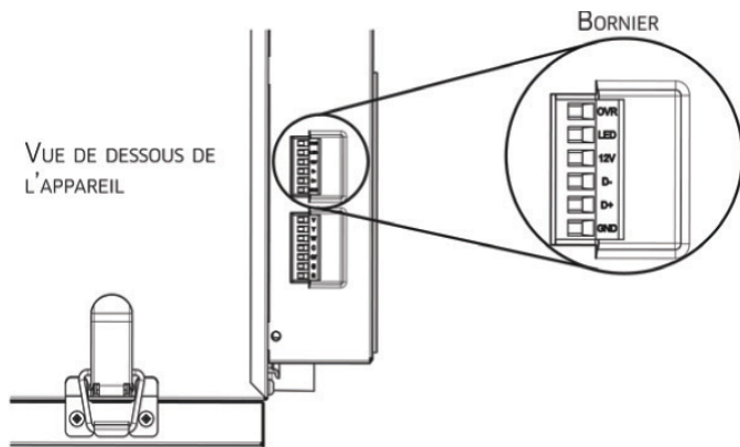
Fig. 16 – Connexion à la Commande Murale
