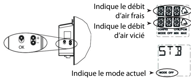
Fig. 22 – Boutons de l'écran LCD
