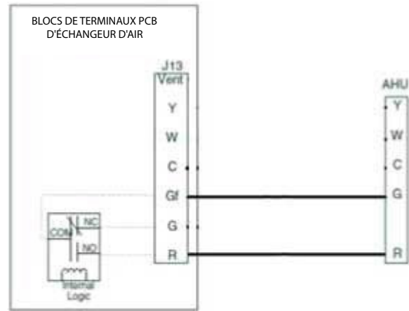
Fig. 20 – Câblage du ventilateur Infinity® / Evolution™ vers l'AHU
