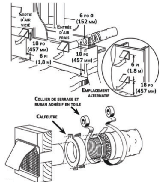
Fig. 12 – Hottes Extérieures
