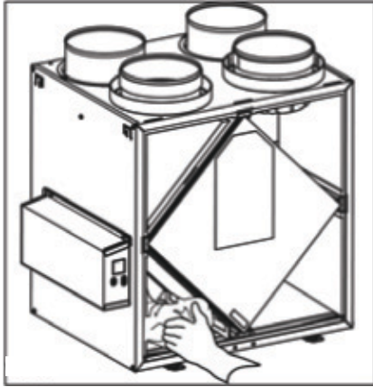
Fig. 26 – Nettoyage Trimestriel
