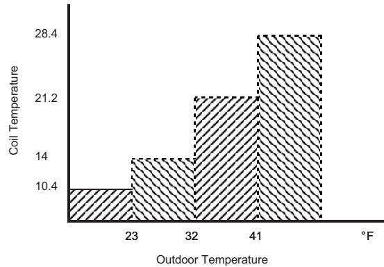
Fig. 23 – Defrost
