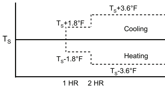
Fig. 26 – SLEEP Mode
