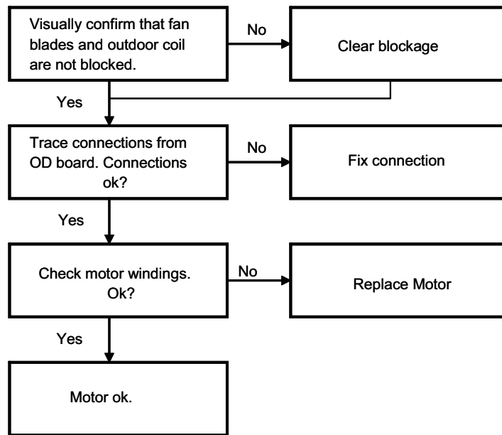
Fig. 38 – Motors
