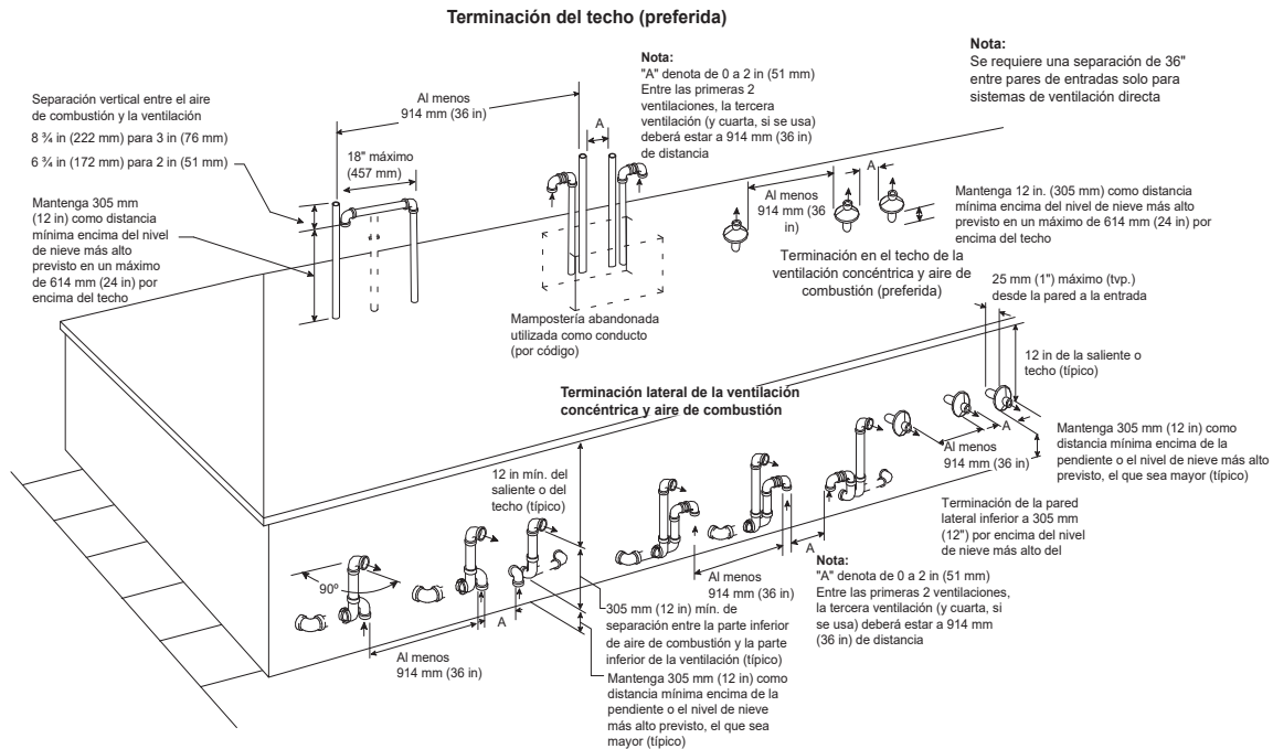
Fig. 40 – Terminación de aire de combustión y de ventilación para sistemas de ventilación directa (2 tuberías)
