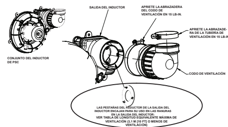
Fig. 53 – Codo de ventilación del inductor
