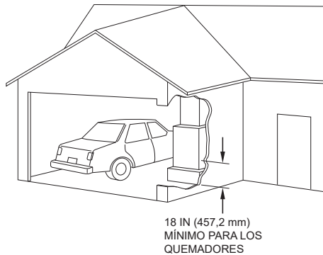
Fig. 5 – Instalación en un garaje
