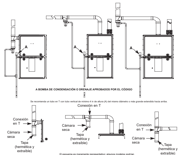
Fig. 51 – Trampa de humedad de admisión de aire A170122ASP de combustión recomendada
