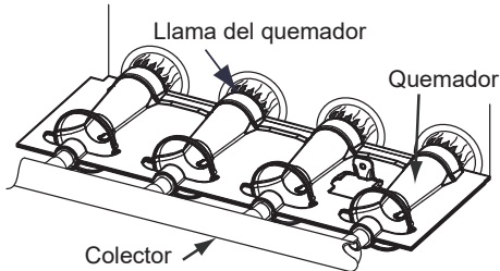
Fig. 62 – Llama del quemador
