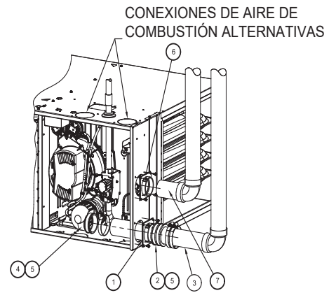
Fig. 57 – Horizontal a la derecha (la apariencia puede variar) Consulte “Notas de opciones de ventilación”
