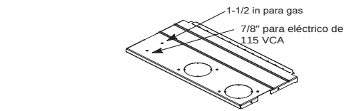
Fig. 31 – Entrada de gas y electricidad alternativa
