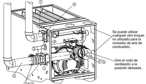
CONFIGURACIÓN CON FLUJO ASCENDENTE HACIA LA IZQUIERDA
