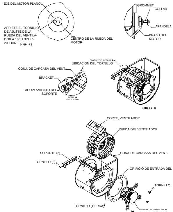
Fig. 66 – Conjunto del ventilador en 040E14--10 y 060E14-12
