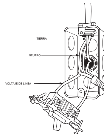
Fig. 36 – Caja eléctrica externa no incluida en la carcasa del calefactor
