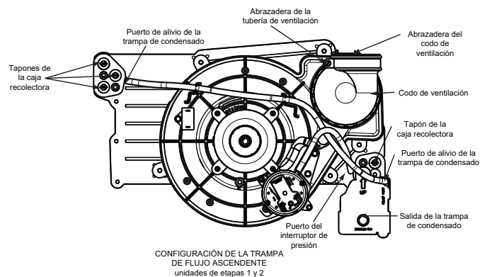
Fig. 8 – Configuración de la trampa en flujo ascendente (La apariencia puede variar)
