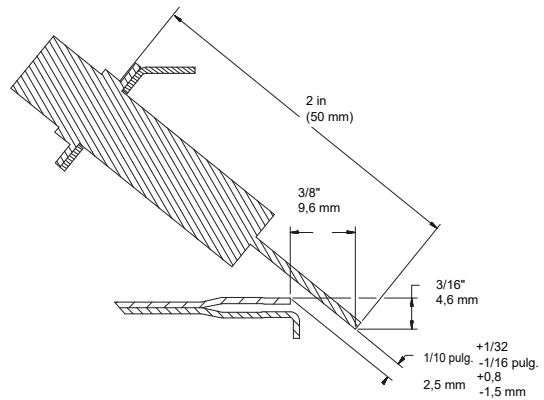
Fig. 70 – Posición del encendedor: vista lateral
