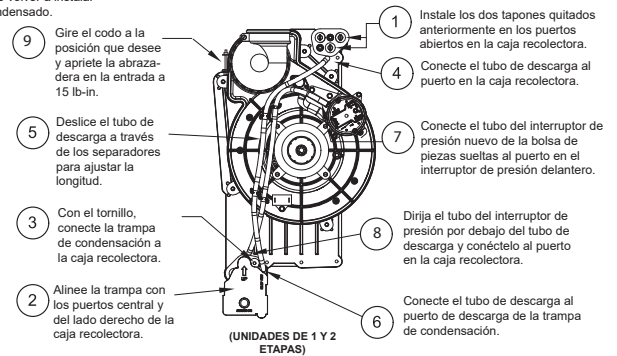
Fig. 11 – Configuración izquierda horizontal de la trampa (La apariencia puede variar)
