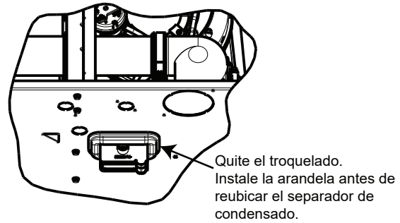
Fig. 18 – Arandela para la trampa de drenaje horizontal
