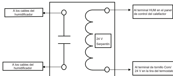
Fig. 38 – Relé de aislamiento, no incluido, para humidificadores con suministro eléctrico interno
