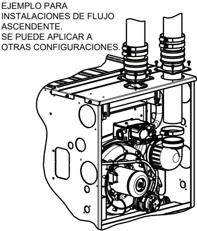
Fig. 44 – Ejemplo de conexión de la tubería de aire de admisión para sistemas de ventilación de polipropileno Ventilación directa/Sistema de 2 tuberías
