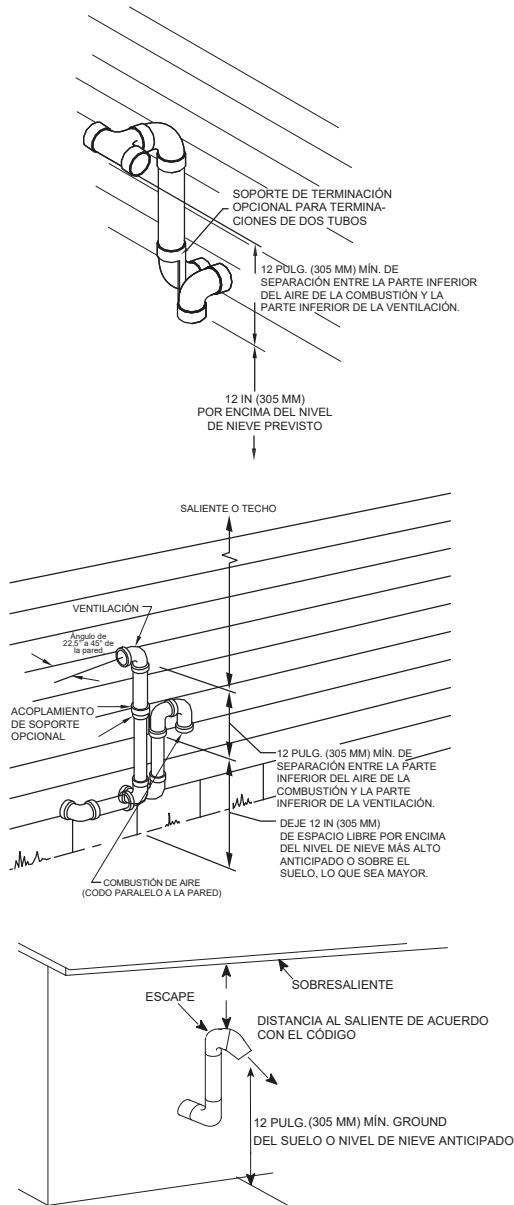
Fig. 49 – Terminación de ventilación en Alberta y Saskatchewan Tamaño de las tuberías de ventilación y aire de combustión
