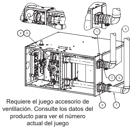
Fig. 56 – Horizontal a la izquierda (la apariencia puede variar) Consulte “Notas de opciones de ventilación”
