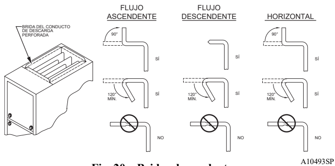
Fig. 20 – Bridas de conductos
