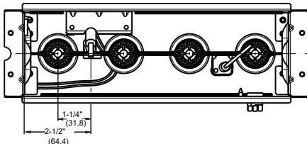
Fig. 69 – Posición del encendedor: vista superior
