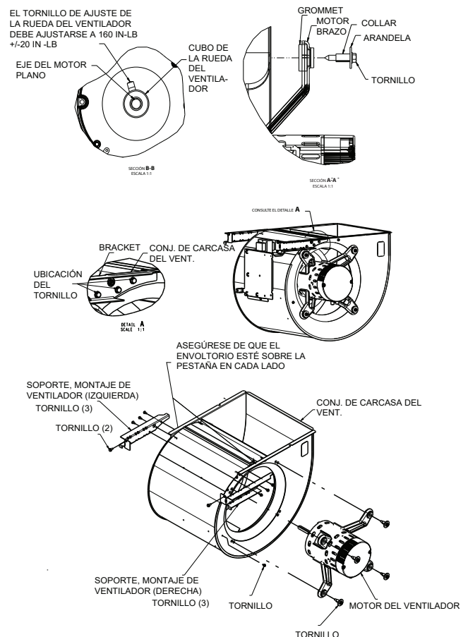
Fig. 67 – Conjunto de ventilador en 100E21--22
