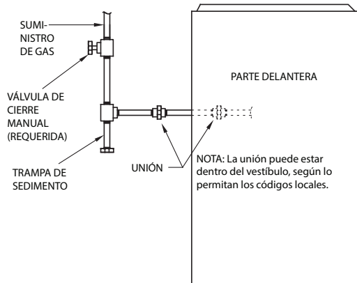
Fig. 32 – Disposición típica de las tuberías de gas
