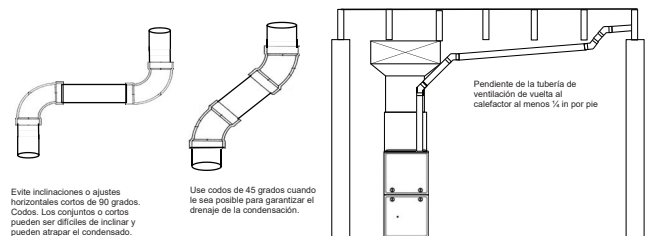
Fig. 52 – Conexiones de ventilación cerca del calefactor
