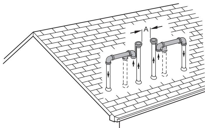
Fig. 48 – Ventilación de tubería y de combustión A96128SP Aire de combustión ventilado
