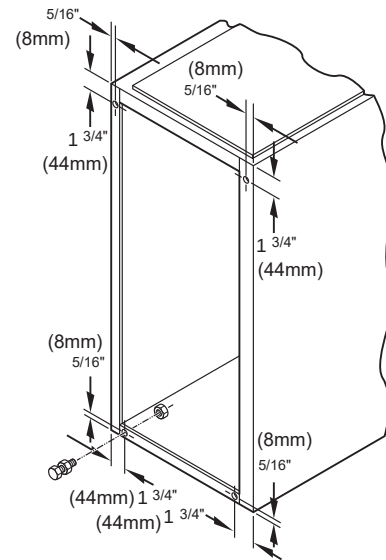
Fig. 29 – Patas niveladoras
