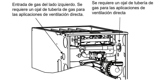
Fig. 30 – Entrada de gas
