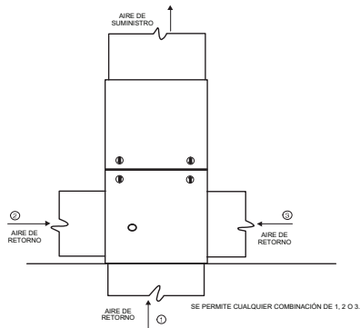
Fig. 21 – Configuraciones y restricciones de aire de retorno de flujo ascendente
