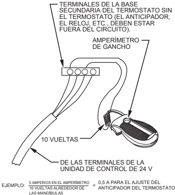
Fig. 64 – Verificación del amperaje con un amperímetro
