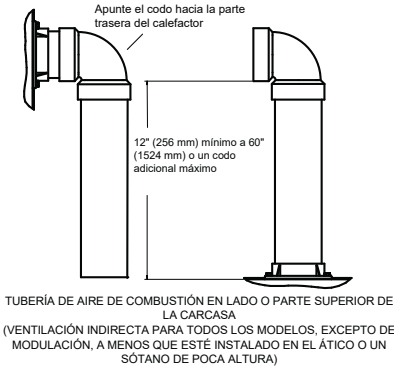
Fig. 45 – Accesorio de tubería de aire de combustión Ventilación indirecta/Sistema de 1 tubería
