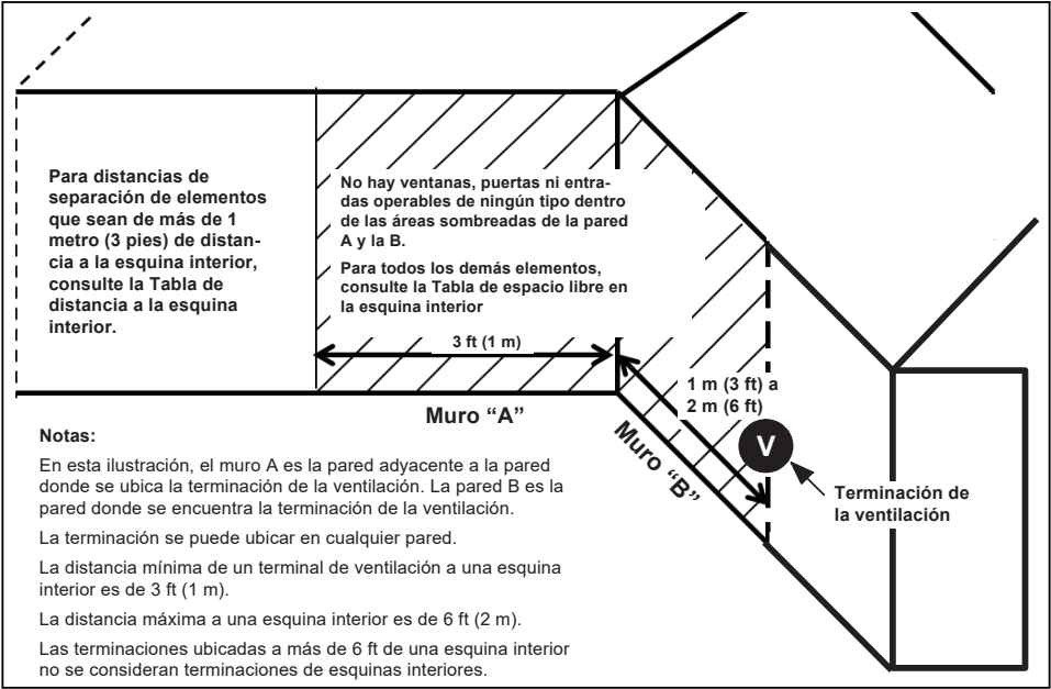
Fig. 46 – Terminación en esquina interna
