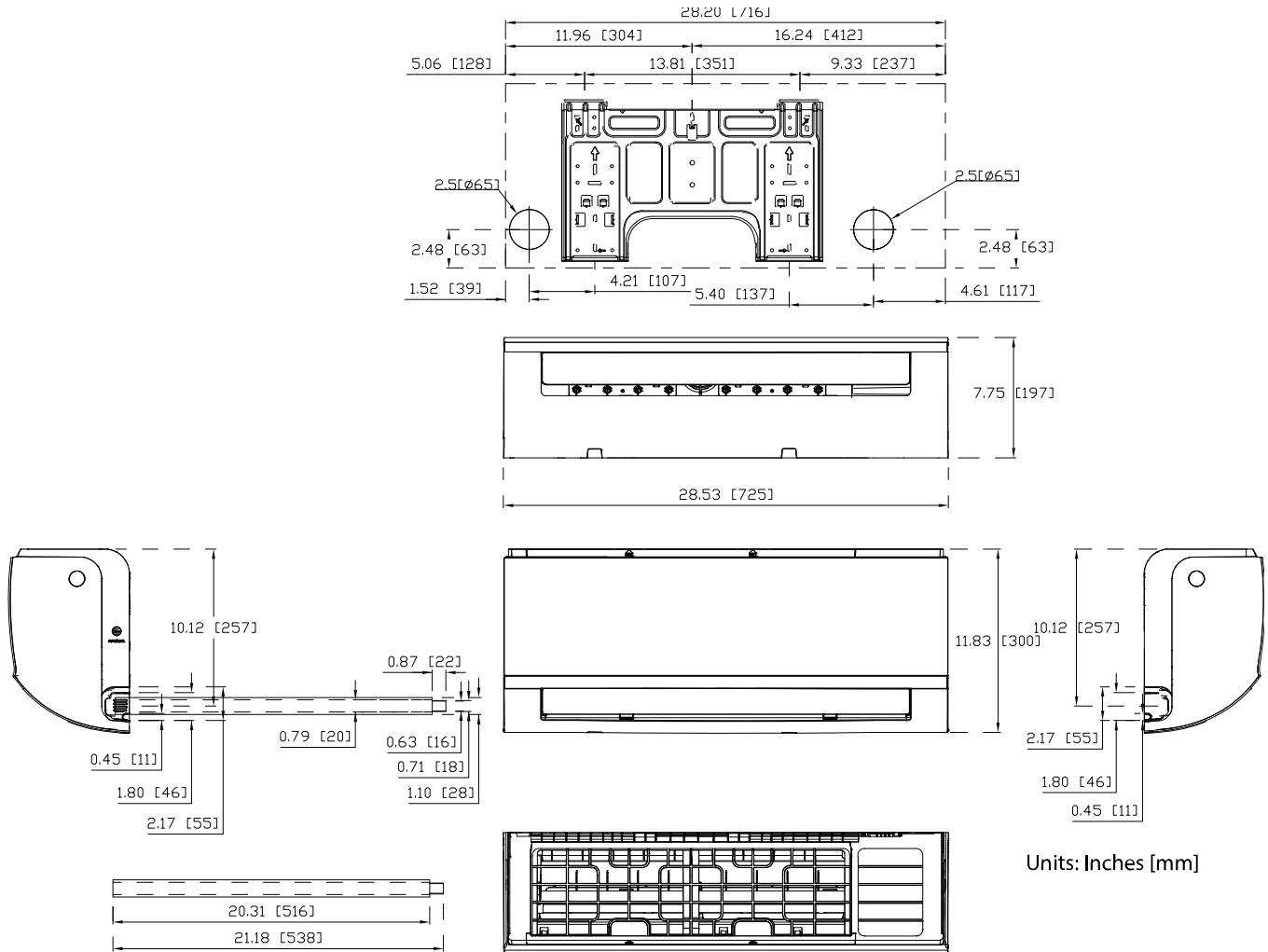
Fig. 5 — Dimensions Size 9K
