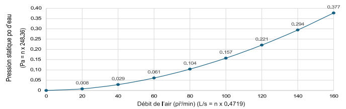
RENDEMENT DU DÉBIT DE L'AIR À L'ALIMENTATION
