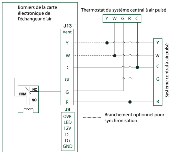
Fig. 21 – Options de Câblage Avec Système Central à Air Pulsé
