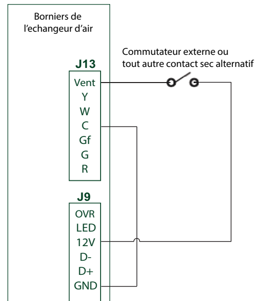
Fig. 19 – Câblage Pour Connexion Par Contact Sec
