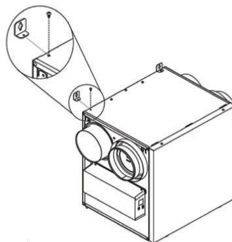
Fig. 3 – Installé au Mur
