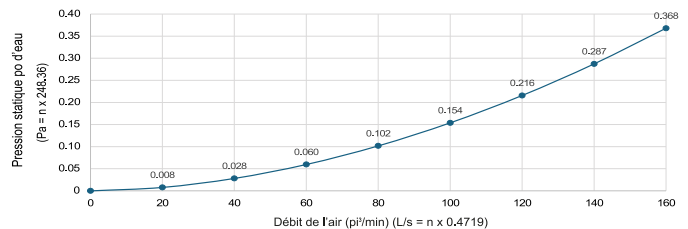
Fig. 13 – Rendement du débit de l'air à l'évacuation
