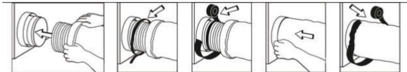
Fig. 15 – Connectez le Conduit à l'Unité
