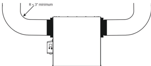
Fig. 16 – Installation Correcte
