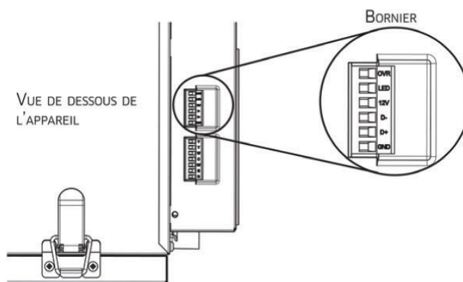
Fig. 18 – Connexion à la Commande Murale
