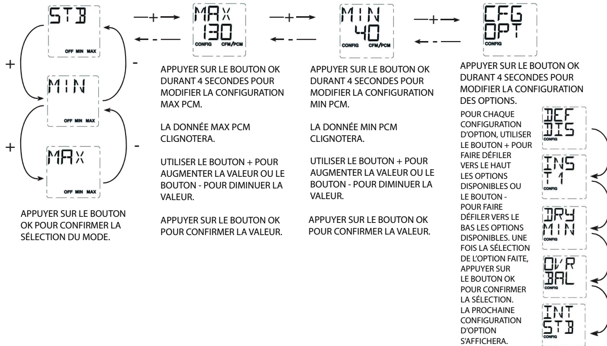
Fig. 25 – Paramètres de Mode et de Configuration
