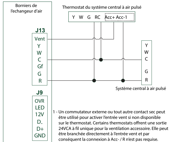
Fig. 19 – Câblage Pour Connexion Par Contact Sec
