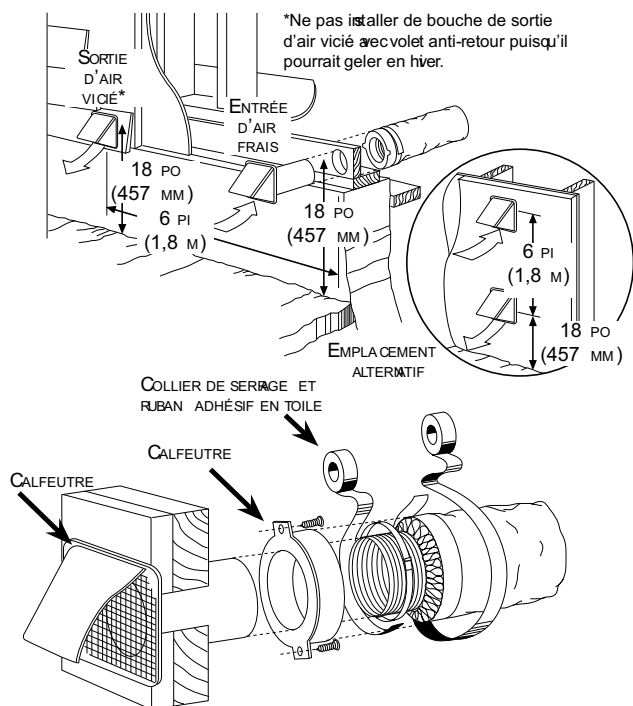
Fig. 14 – Hottes Extérieures
