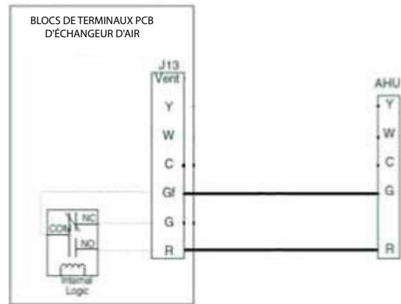
Fig. 22 – Câblage du ventilateur Infinity® / Evolution™ vers l'AHU
