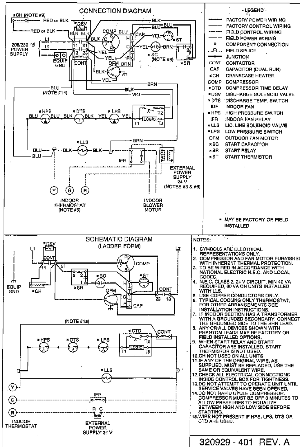
Fig. 2—597C060 208/230v, 1 Phase, 60 Hertz
