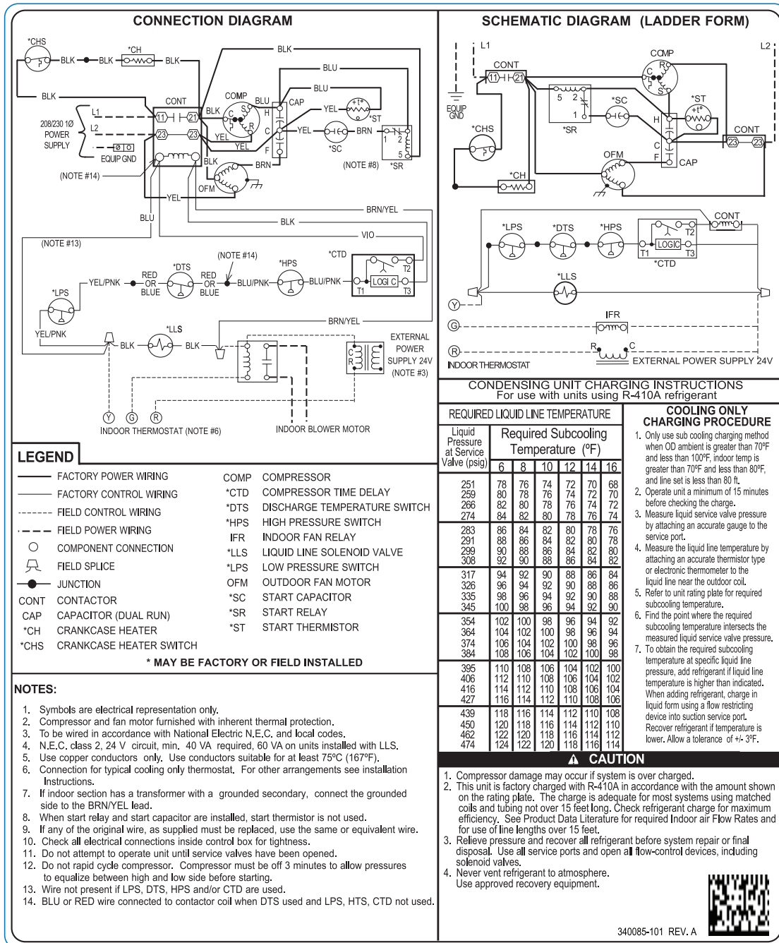
Fig. 1 – 24ACC618-48, 208/230-1
