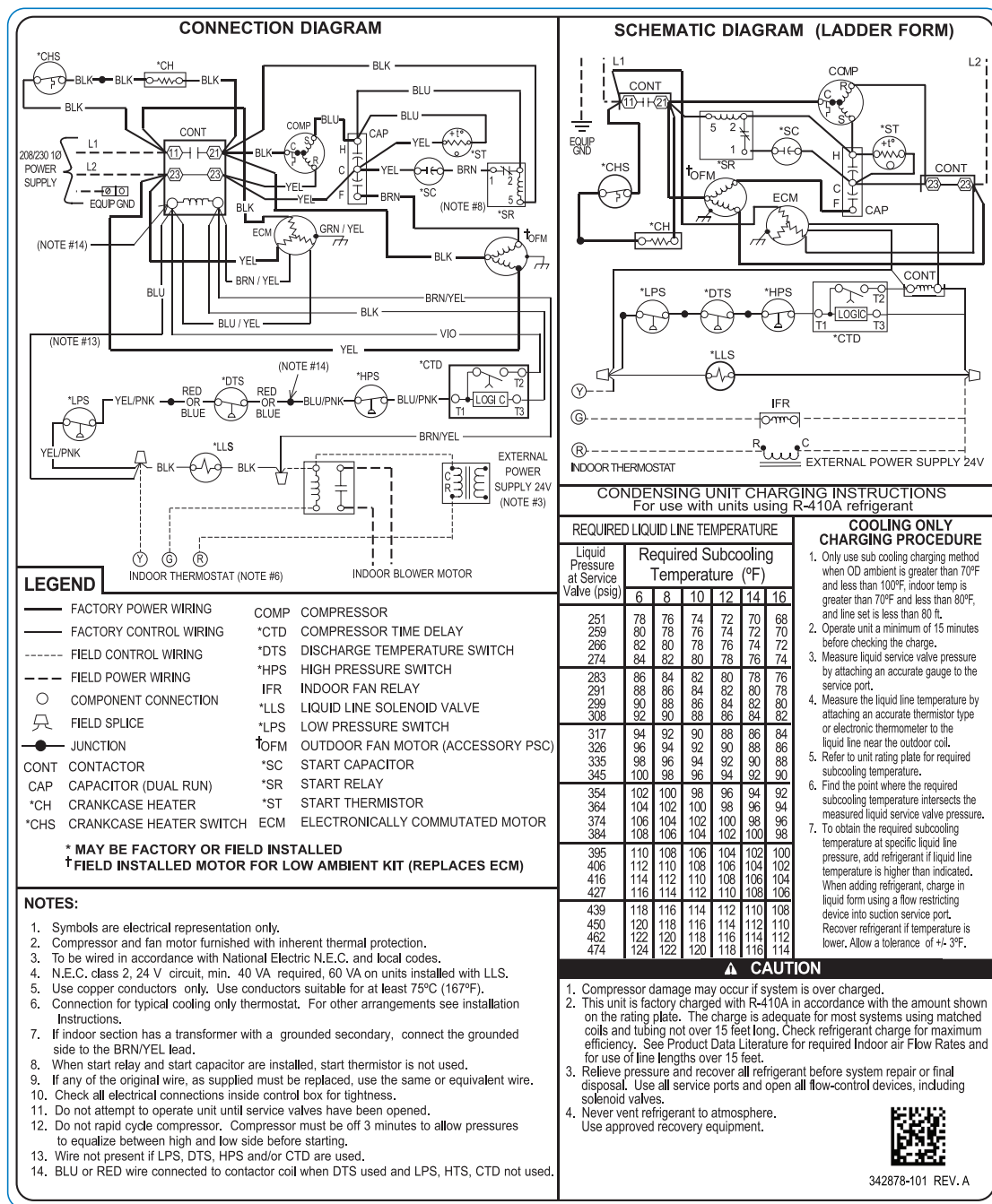
Fig. 1 – 24ACC660, 208/230-1
