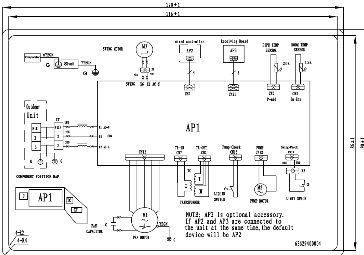
Fig. 31 – Wiring Diagram Cassette 24k
