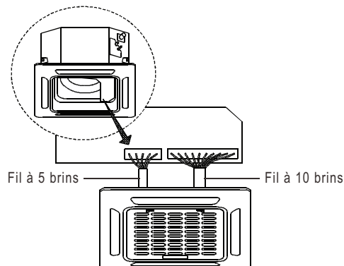
Figure 23 – Branchement des deux faisceaux de câblage
