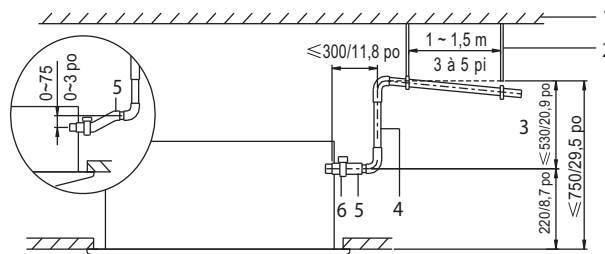
Figure 14 – Installation du flexible d'évacuation
