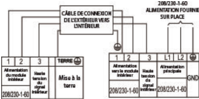
Unité intérieure 12K à 30K 208-230V Unité extérieure 12K à 30K 208-230V
