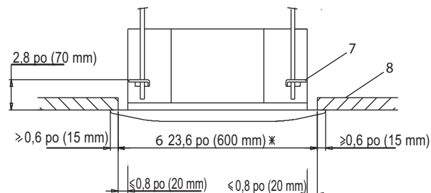
Figure 6 – Perçage de trous
