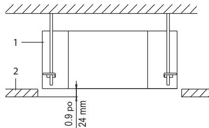
Figure 7 – Perçage de trous
