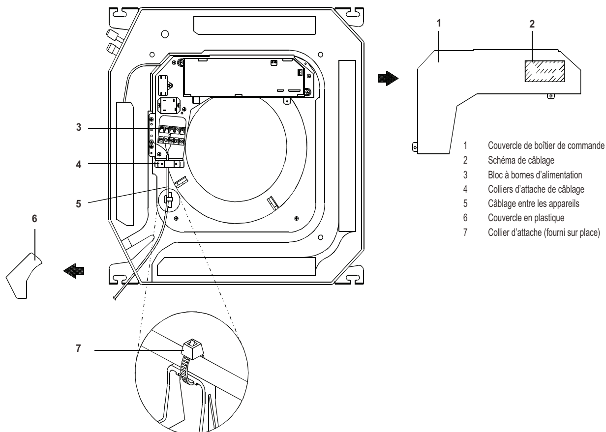
Figure 17 – Boîtier de câblage et de commande
