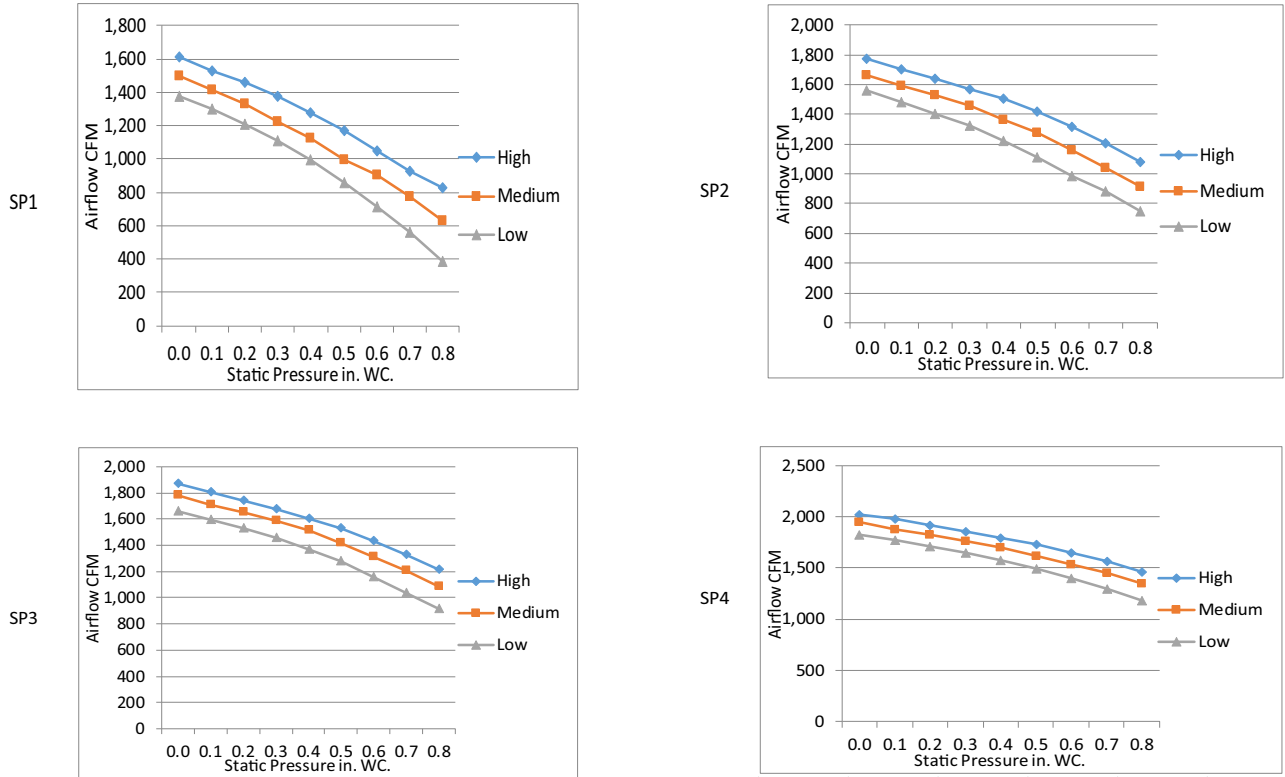
Fig. 11 — Fan Performance - 48K
