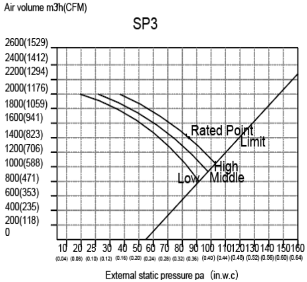
Fig. 16 — Fan Performance - DLFSDAH24XAK
