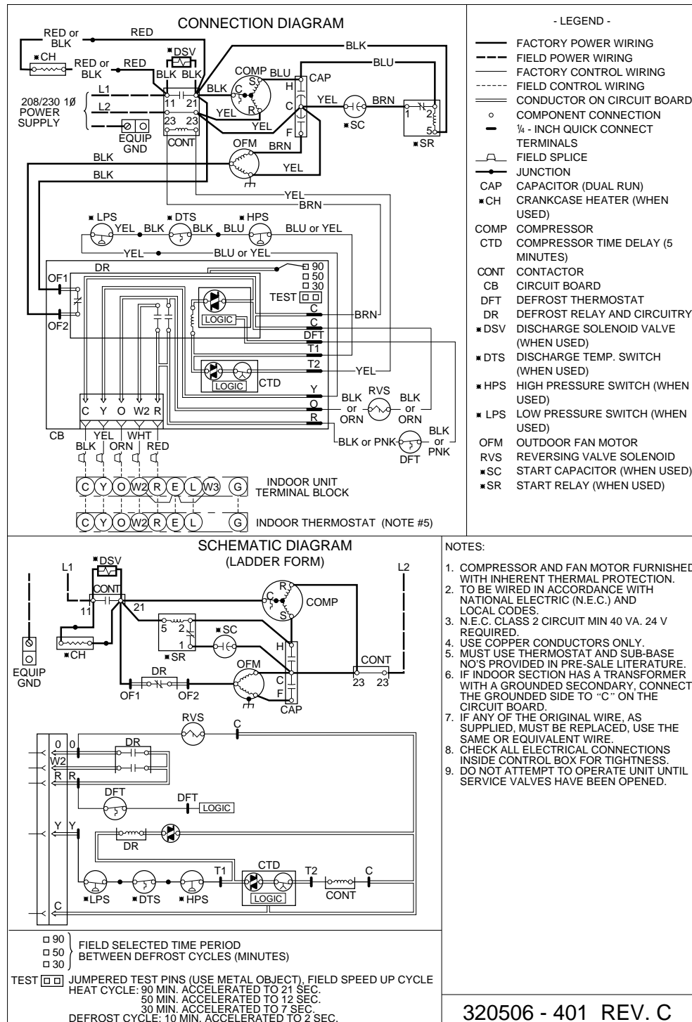
Fig. 1—38BY018-048 208/230v, 1 Phase, 60 Hertz
