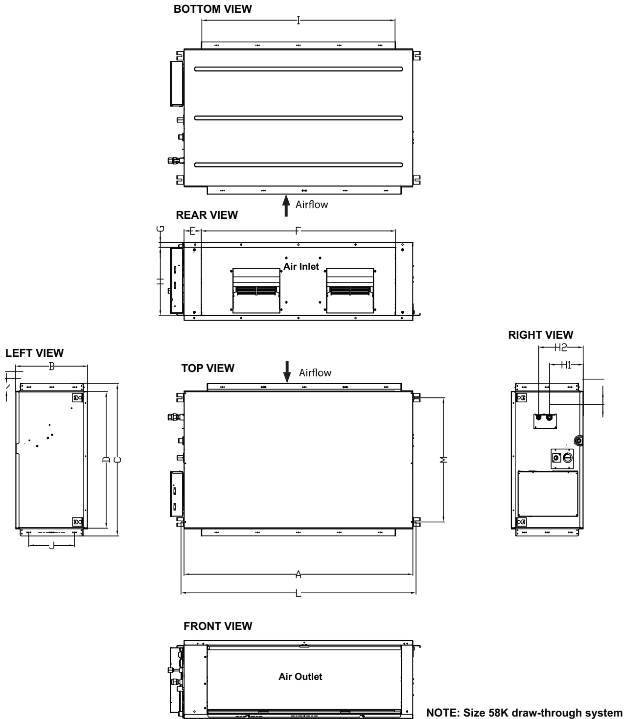
Fig. 6 — Indoor Unit Size 58K
