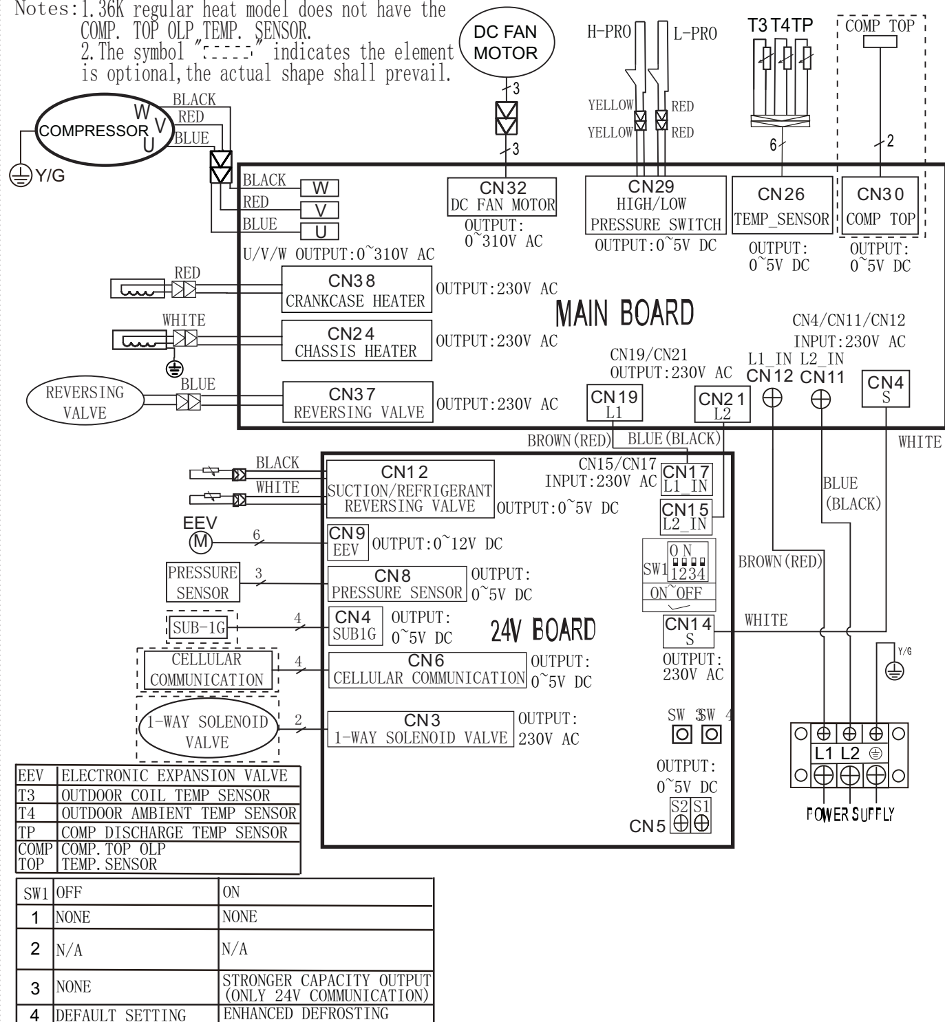
Fig. 18 – 36K Wiring Diagram
