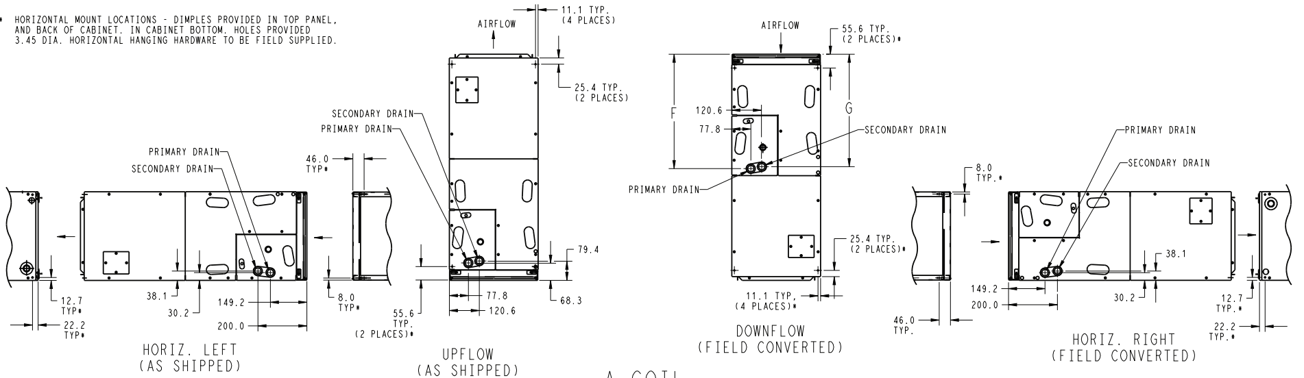
Fig. 4 – FX4DNF - Metric
