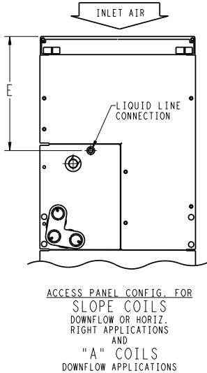
Fig. 3 – FX4DNF - Metric
