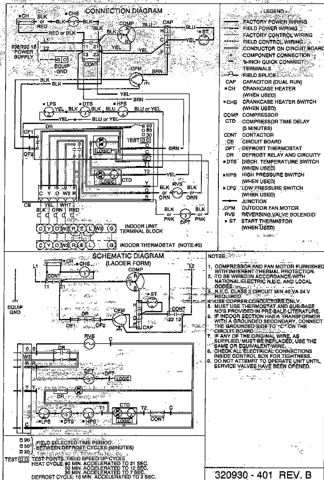
Fig. 2—693C060 208/230v, 1 Phase, 60 Hertz
