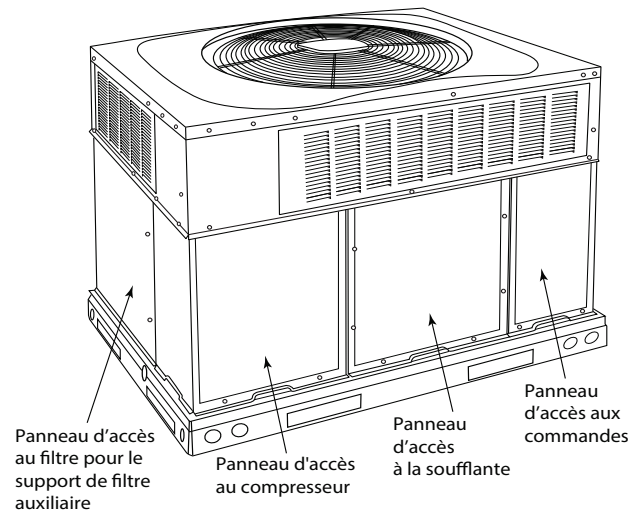
Fig. 2 – Panneau d'accès de l'appareil
