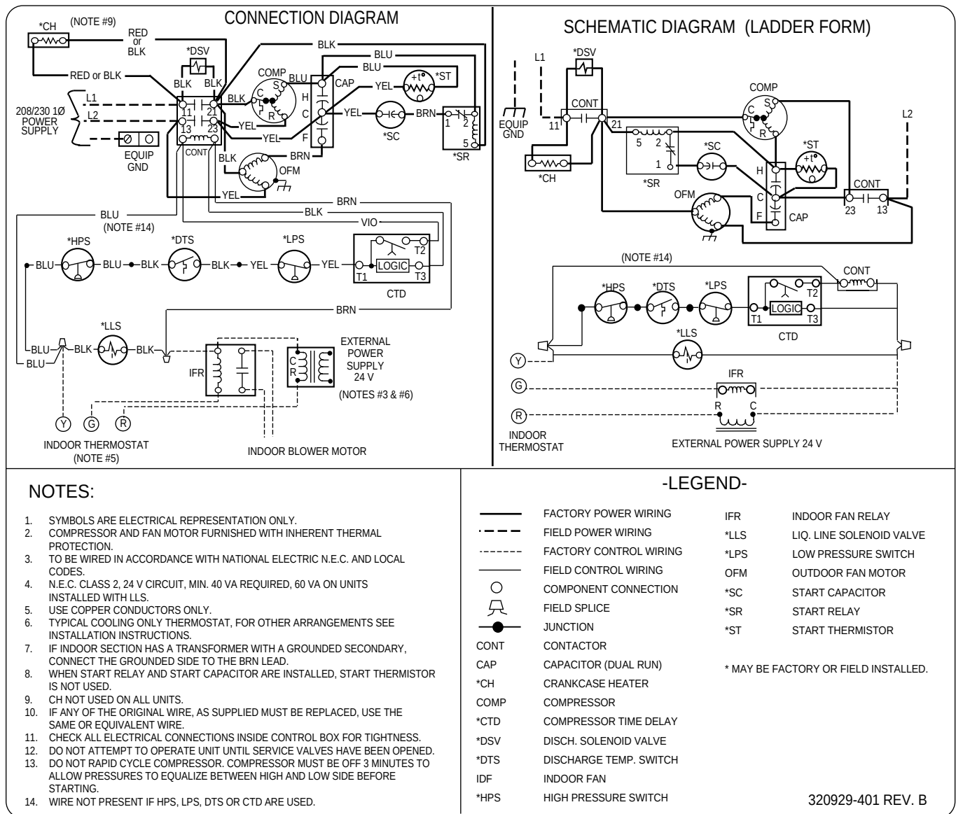
Fig. 2—38TRA060(1,3); 208/230v, 1 Phase, 60 Hertz
