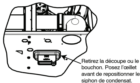
Fig. 18 – Œillet de siphon d'évacuation horizontal
