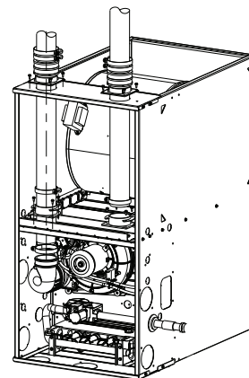
CONFIGURATION À DROITE À TIRAGE DESCENDANT
