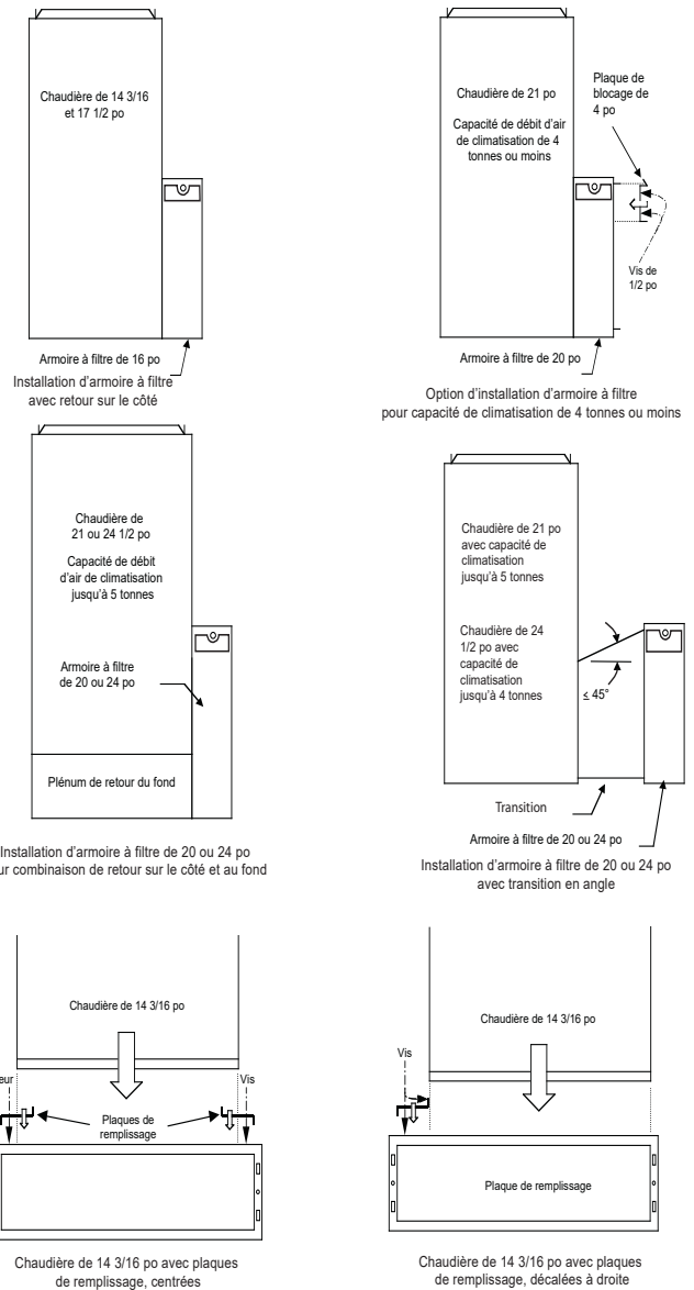
Fig. 27 – Accessoire pour armoire à média filtrant en option
