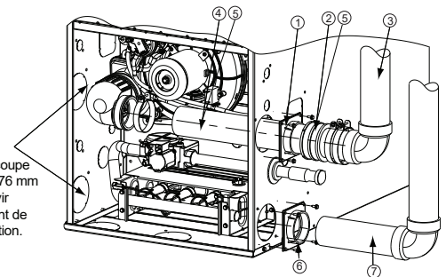
CONFIGURATION À DROITE À TIRAGE DESCENDANT
