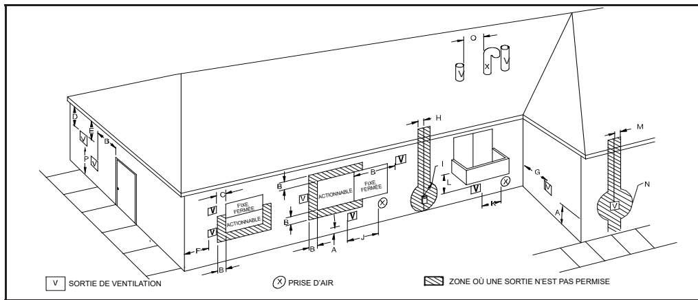
Fig. 42 – Dégagement de sortie à ventilation directe
