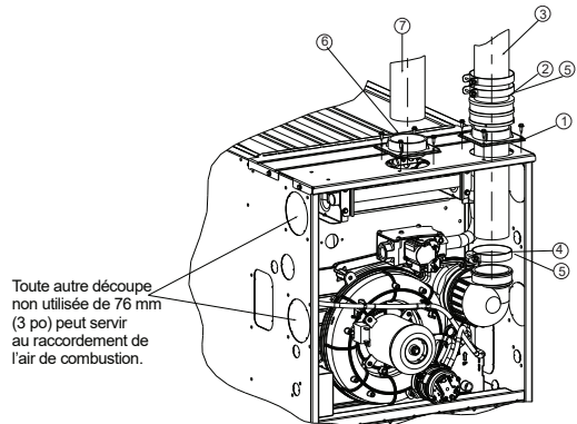
VENTILATION VERTICALE À TIRAGE ASCENDANT Fig. 54 – Configurations de siphon à tirage ascendant (l'apparence peut varier)
