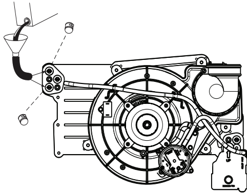
CONFIGURATION DE SIPHON À TIRAGE ASCENDANT PRINCEPS A1 ET A3 PHASES
