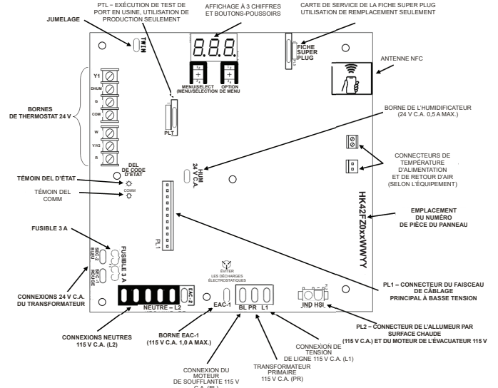
Fig. 38 – Exemple de panneau de commande de chaudière à une phase
