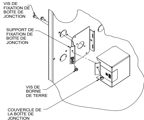
Fig. 35 – Installation d'une boîte de jonction (le cas échéant)
