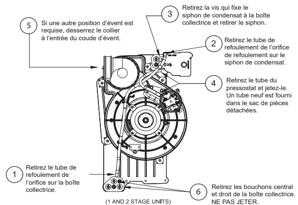
Fig. 10 – Configuration de siphon horizontal à droite (l'apparence peut varier)
