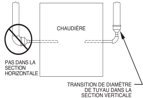
Fig. 49 – Sortie de ventilation pour l'Alberta et la Saskatchewan
