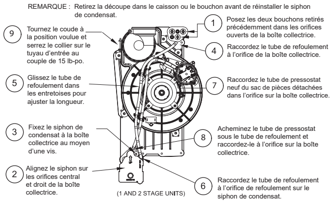
Siphon en configuration horizontale à gauche
