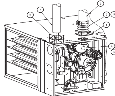
CONFIGURATION HORIZONTALE À GAUCHE ET VENTILATION VERTICALE
