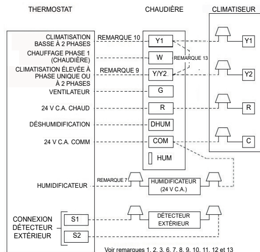
Appareil de chauffage à un étage avec climatiseur
