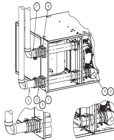
CONFIGURATION HORIZONTALE À DROITE ET VENTILATION À GAUCHE
