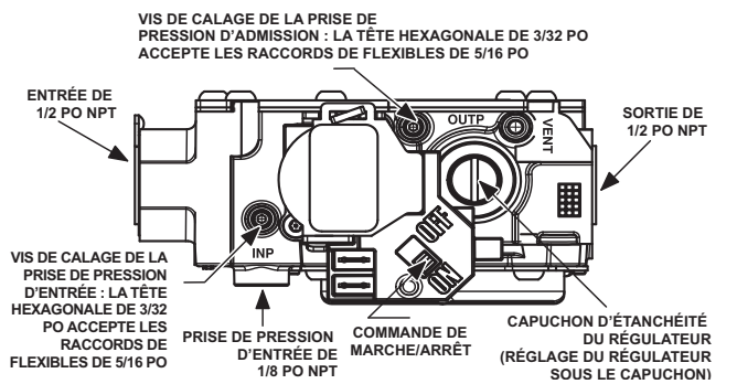
Fig. 64 – Soupape de gaz avec orifices de pression
