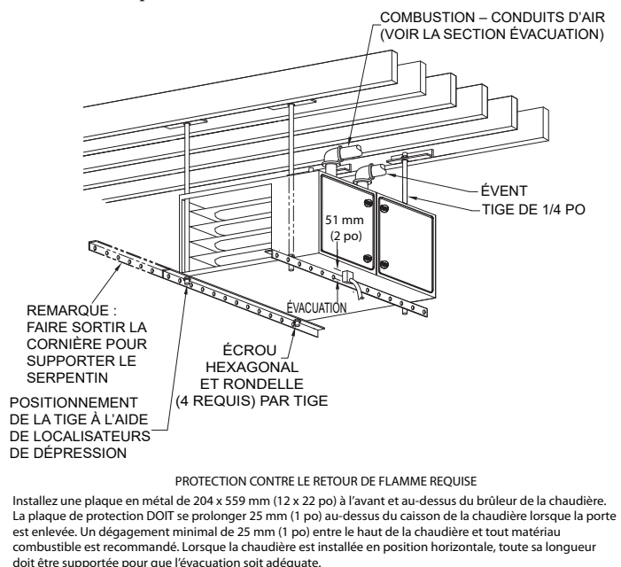
Fig. 29 – Installation de chaudière suspendue
