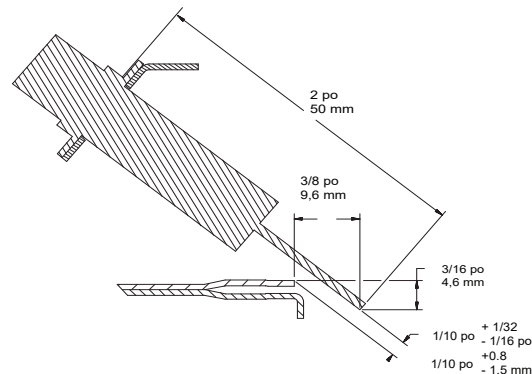
Fig. 69 – Position de l'allumeur – vue latérale
