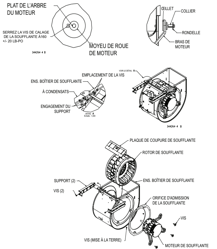
Fig. 66 – Ensemble de soufflante
