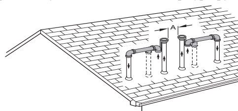
Fig. 46 – Sortie d'évacuation et de combustion
