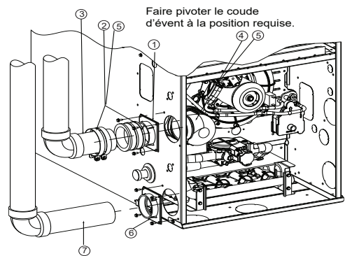
CONFIGURATION À GAUCHE À TIRAGE DESCENDANT
