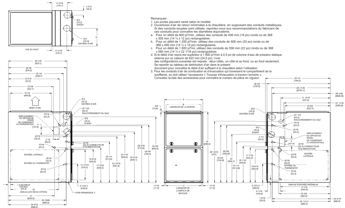
Fig. 1 – Schéma des cotes Tableau 1 – Dimensions
