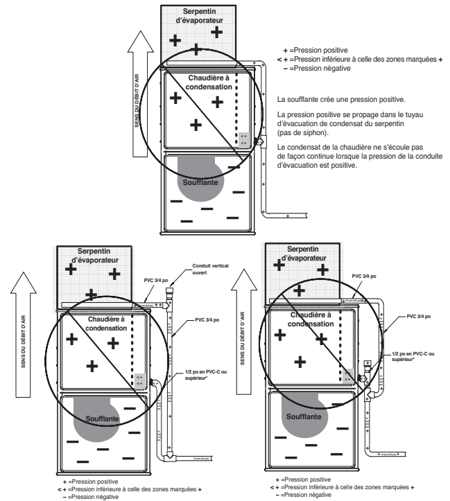
Fig. 13 – Exemple de fixation au tuyau d'évacuation sur place (non autorisée)
