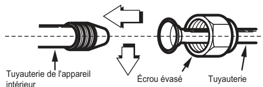
Fig. 18 — Alignez le centre du tuyau
