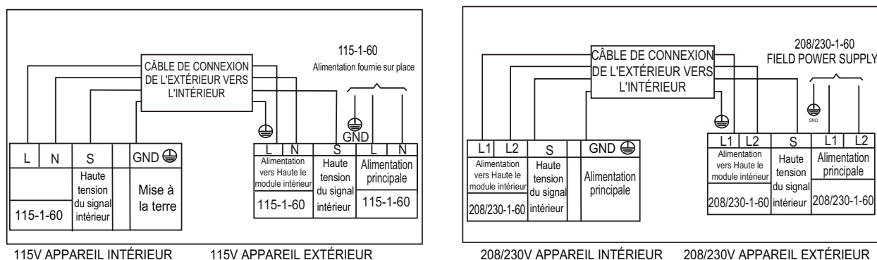
Fig. 12 — Schémas de raccordement
