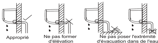
Fig. 20 — Installation appropriée du flexible d'évacuation
