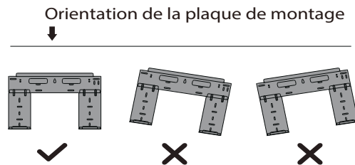
Fig. 9 — Orientation de la plaque de montage
