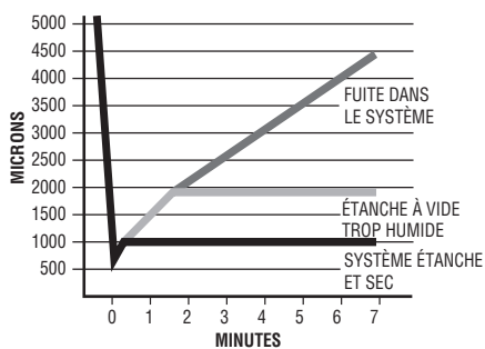
Figure 4 – Schéma du vide poussé
