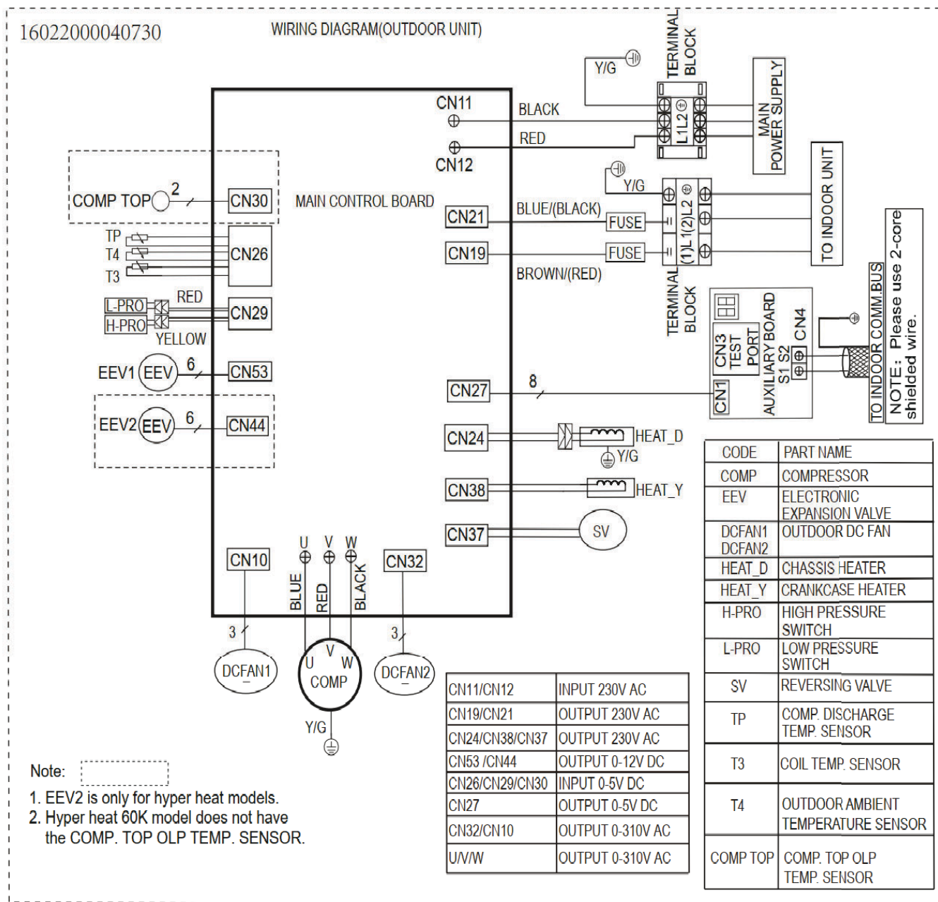
Fig. 8 – 48K / 58K Wiring Diagram
