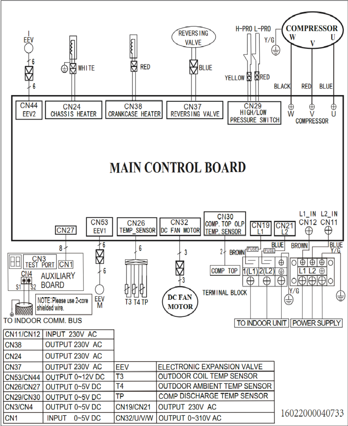
Fig. 7 – 36K Wiring Diagram
