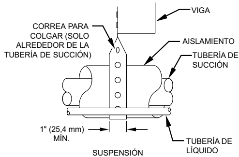
Fig. 1 – Instalación de tuberías
