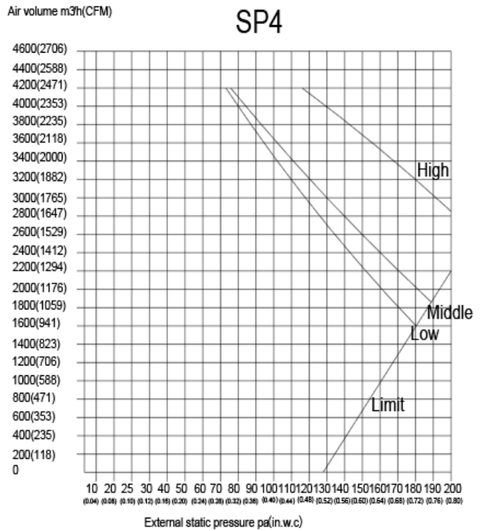
Fig. 19 — Fan Performance - DLFLDAH58XAK
