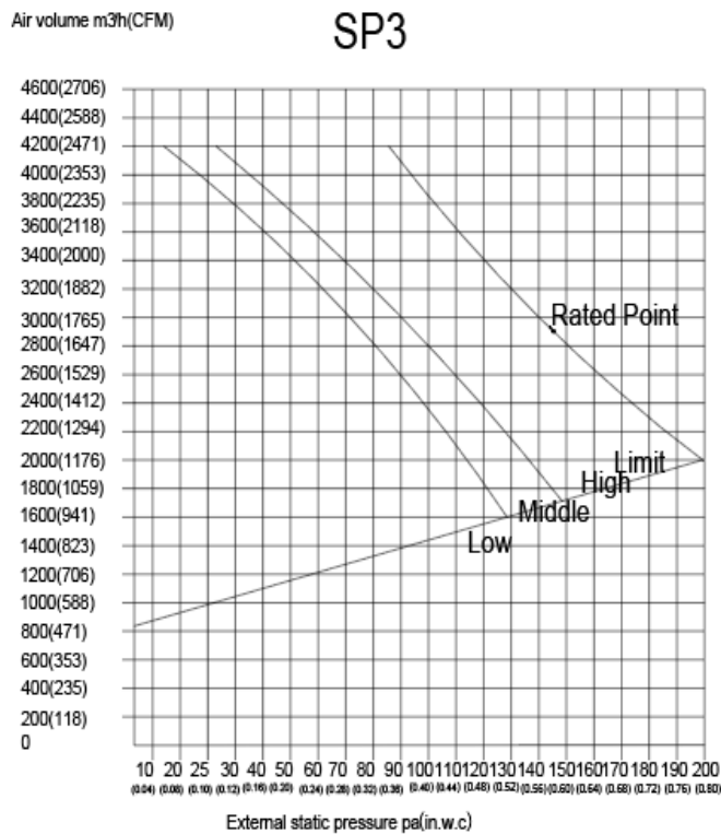
Fig. 19 — Fan Performance - DLFLDAH58XAK
