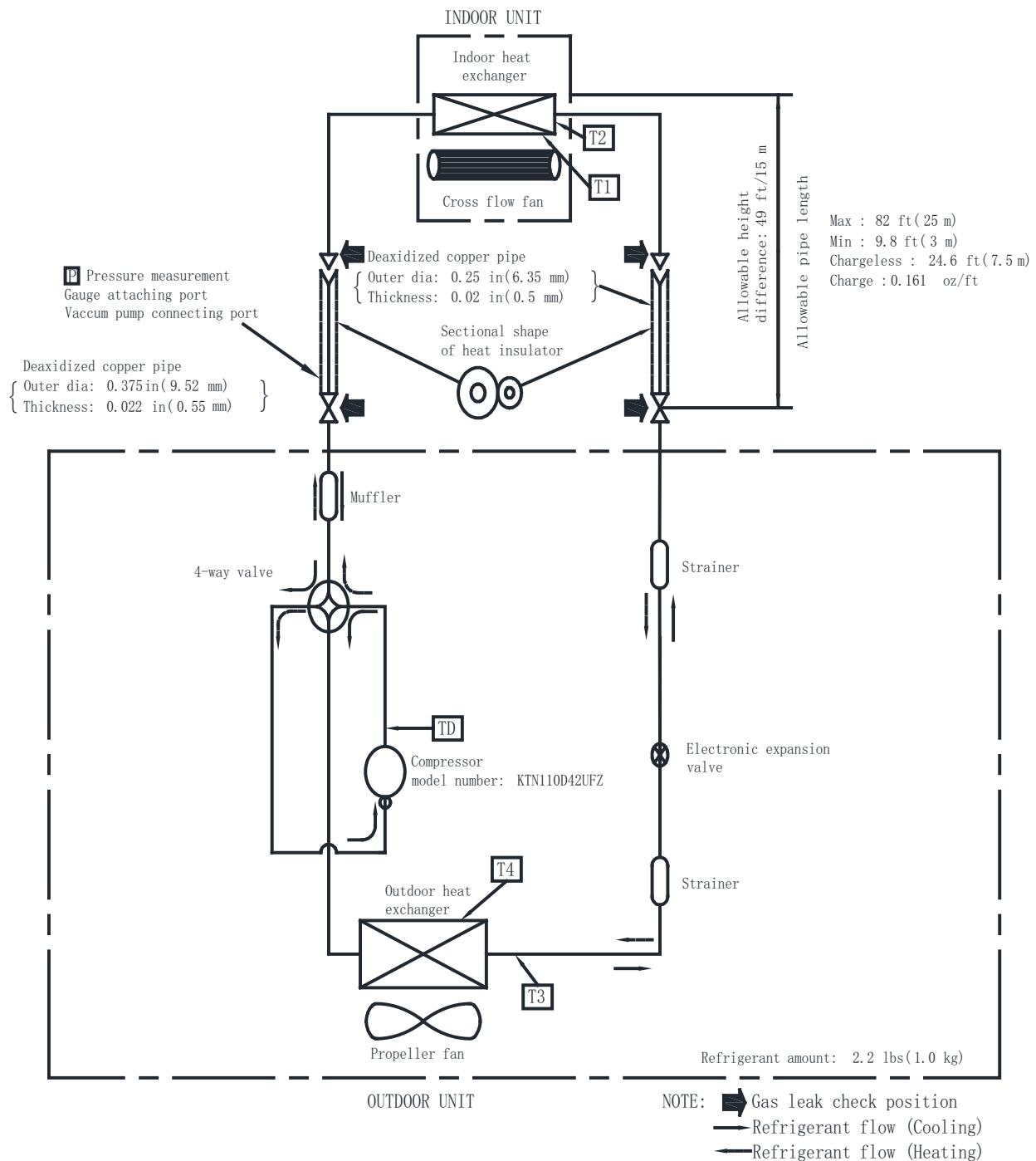
Fig. 16 —Size 9K/12K
