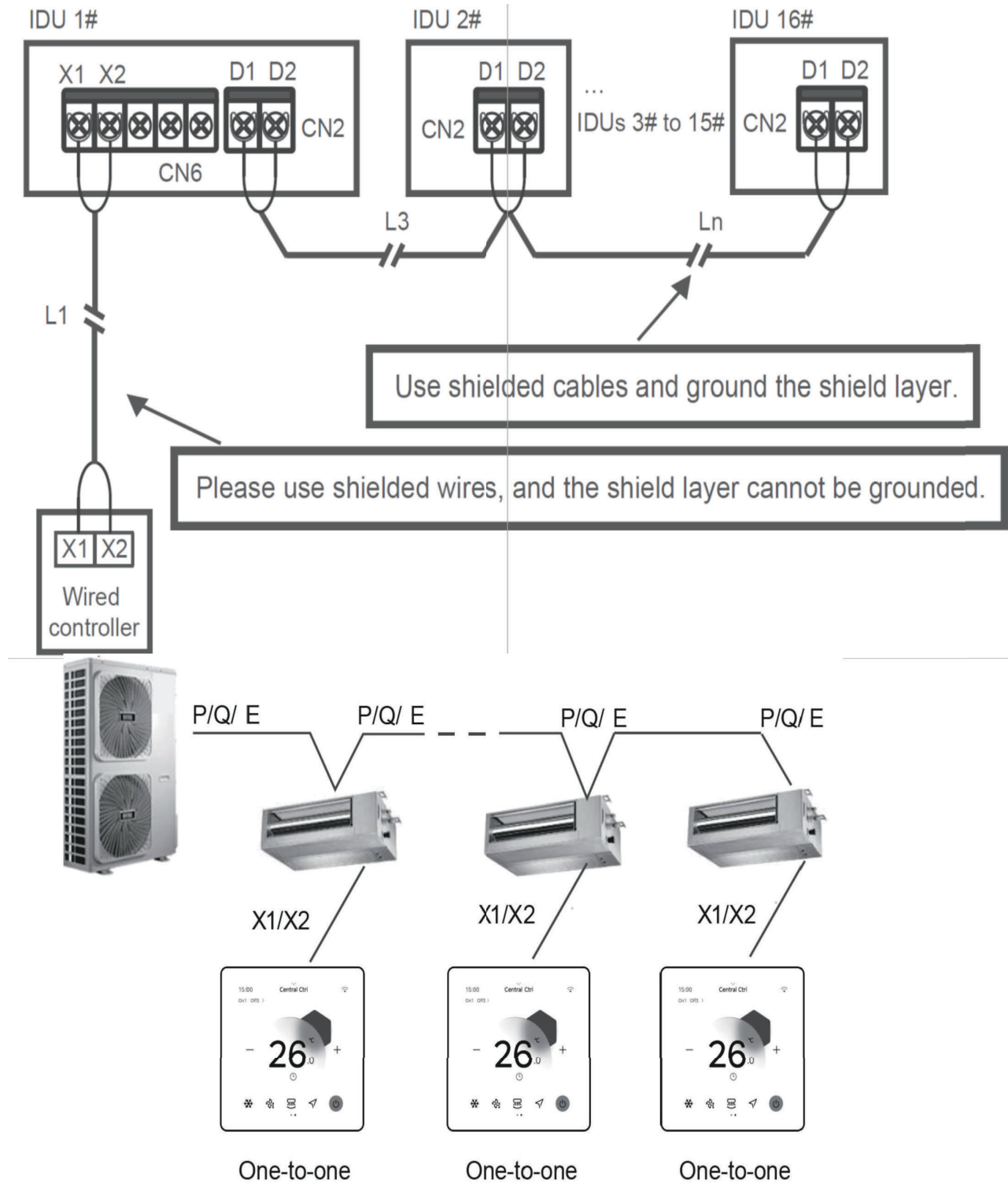
Fig. 3 – Wiring Diagram
