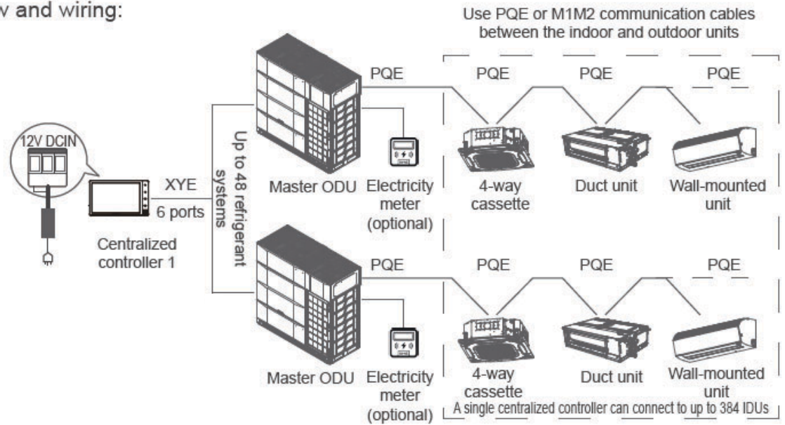
Fig. 3 – Wiring Diagram
