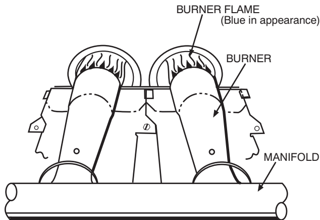
Fig. 9 - Monoport Burner
