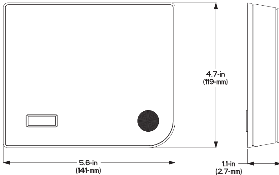
Fig. 1 - Unit Dimensions
