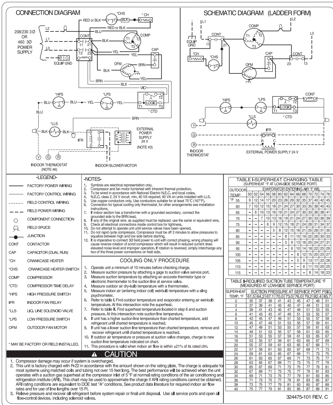
Fig. 1—PA10 036, 048, 060
