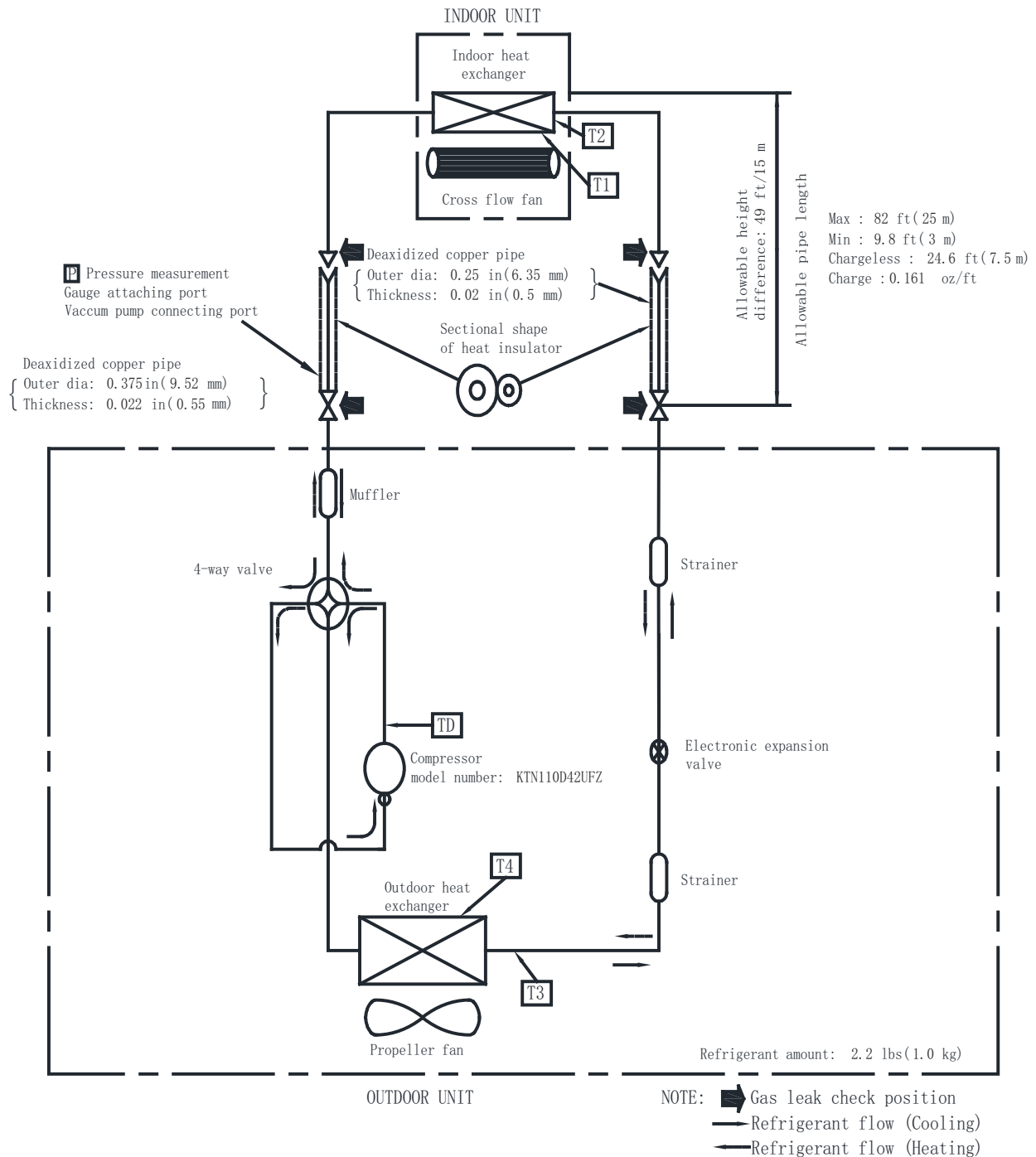
Fig. 16 —Size 9K/12K
