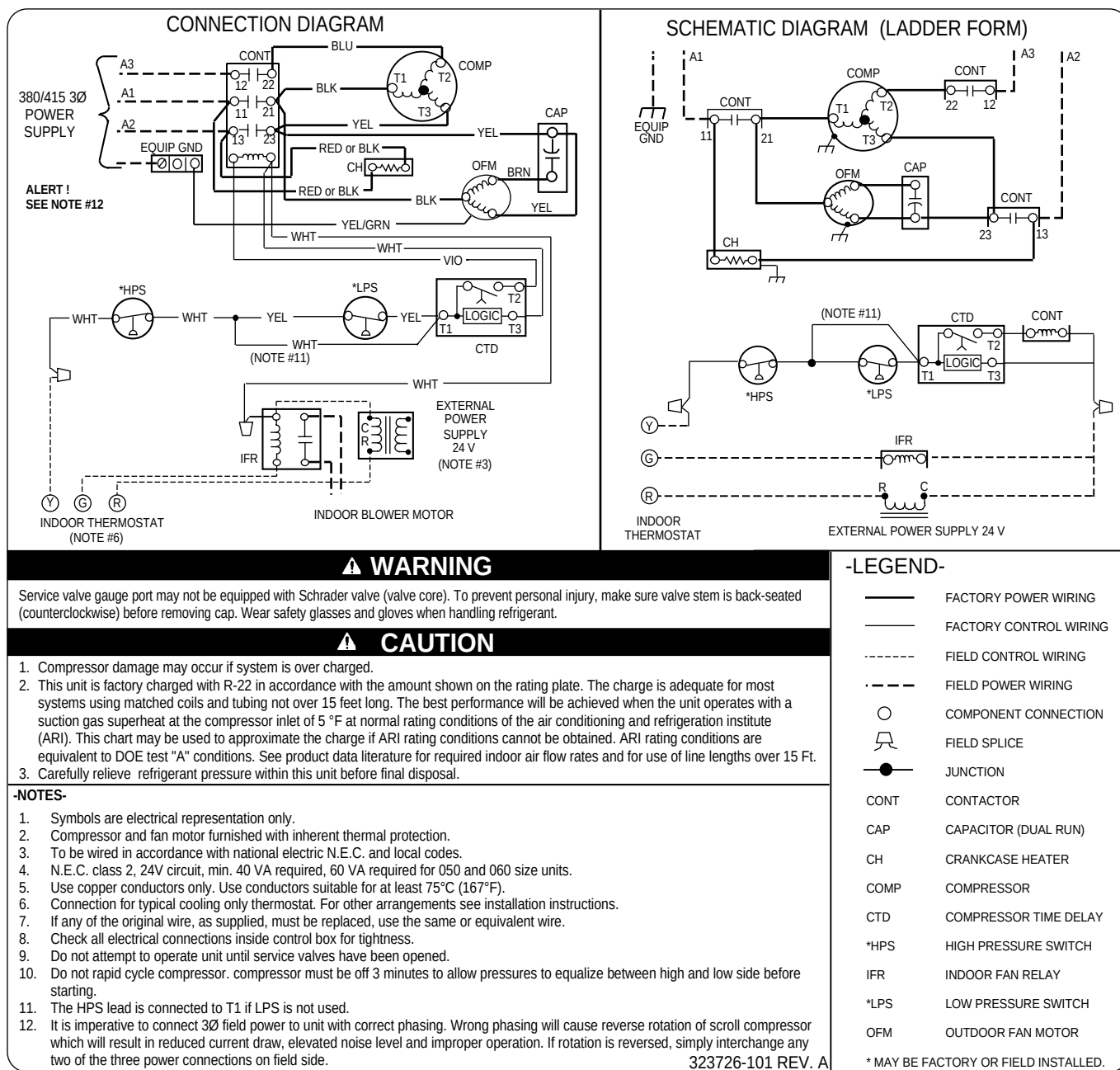
Fig. 2—38TUA036, 048, 060 400v, 3 Phase, 50 Hertz
