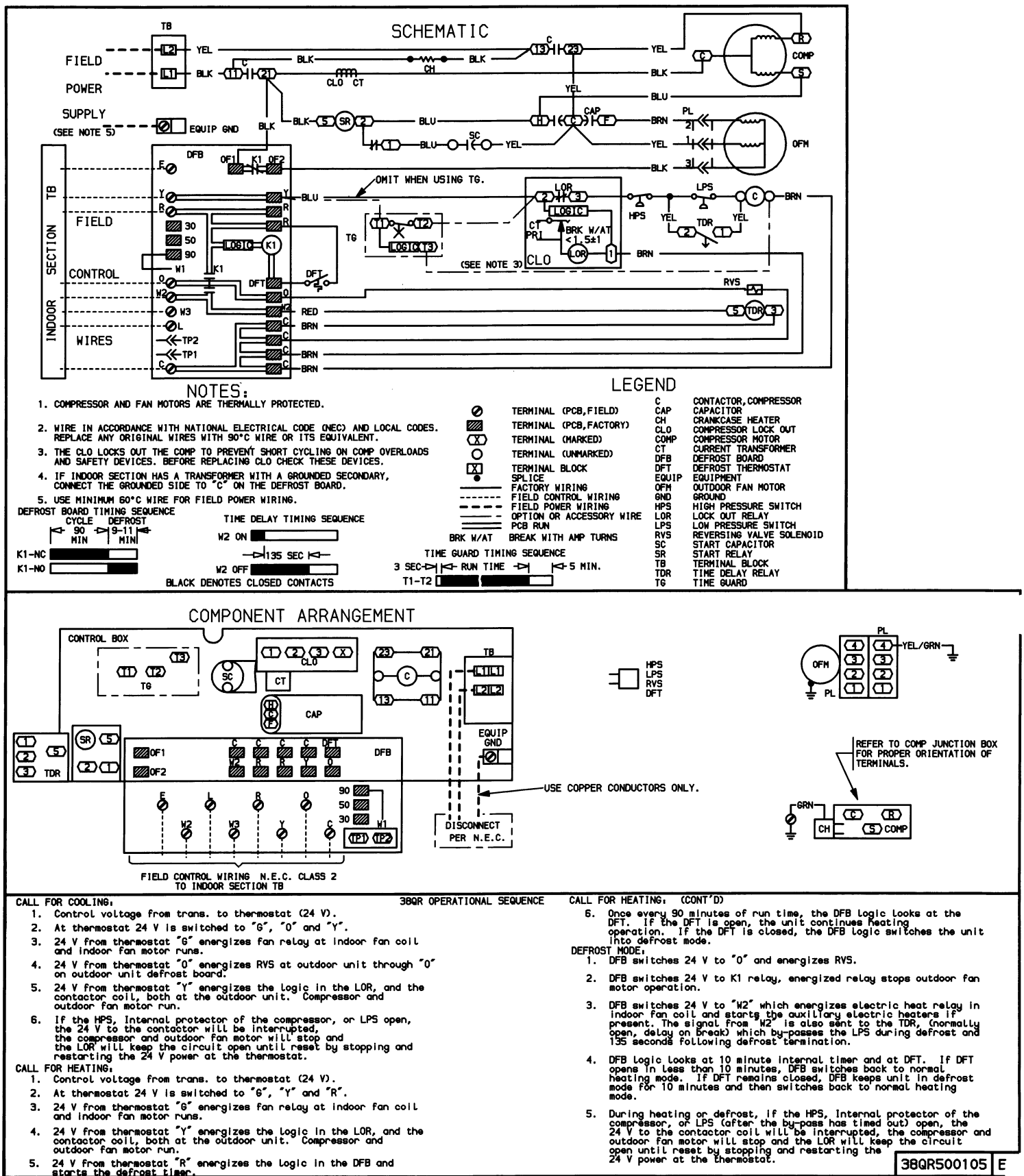
Fig. 9—208/230 Volt, 1 Phase, 60 Hertz (38QR)
