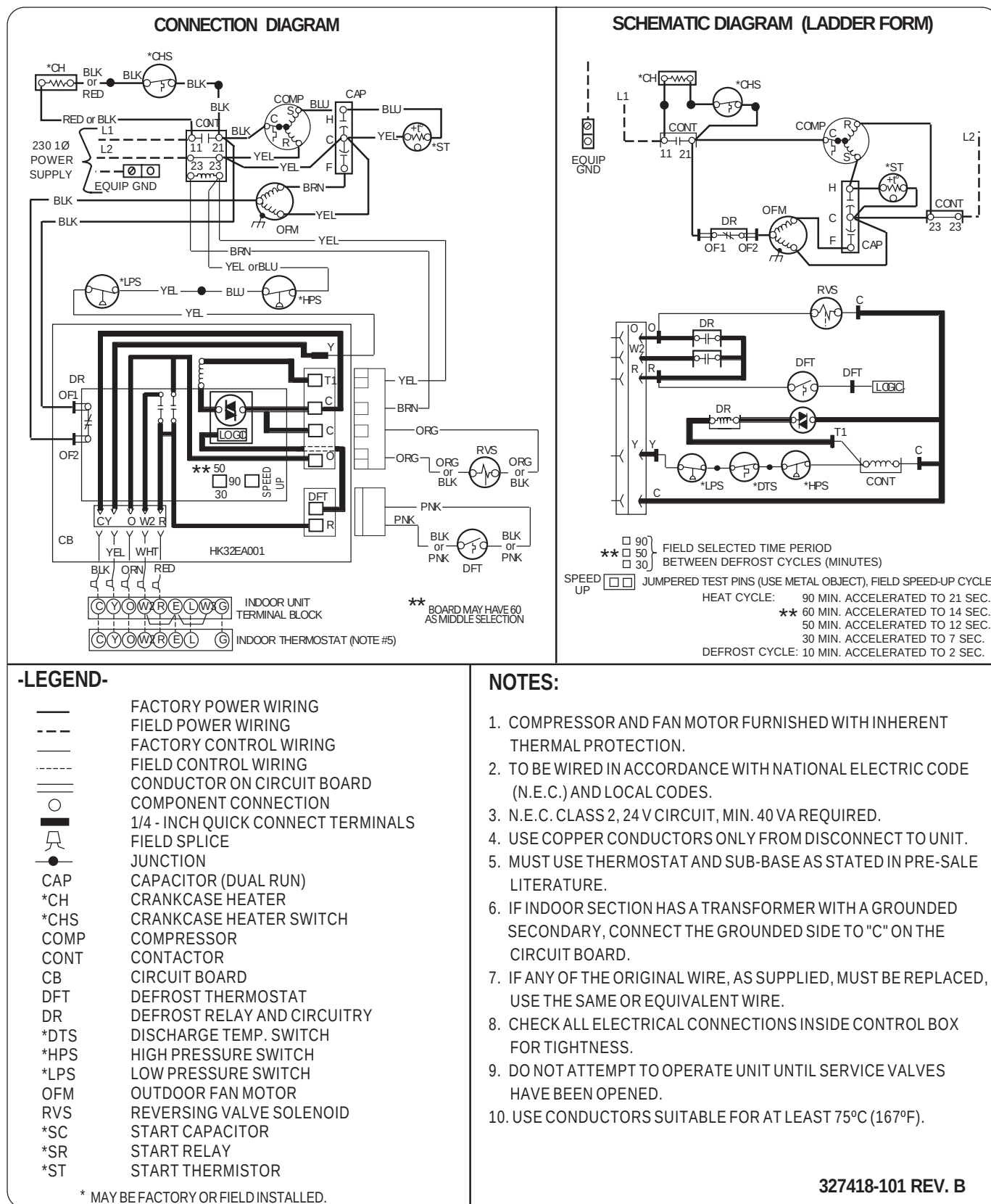
Fig. 9—Label Wiring 327418-101
