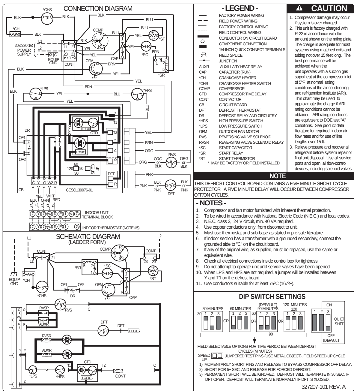
Fig. 1—Label Wiring 327207-101
