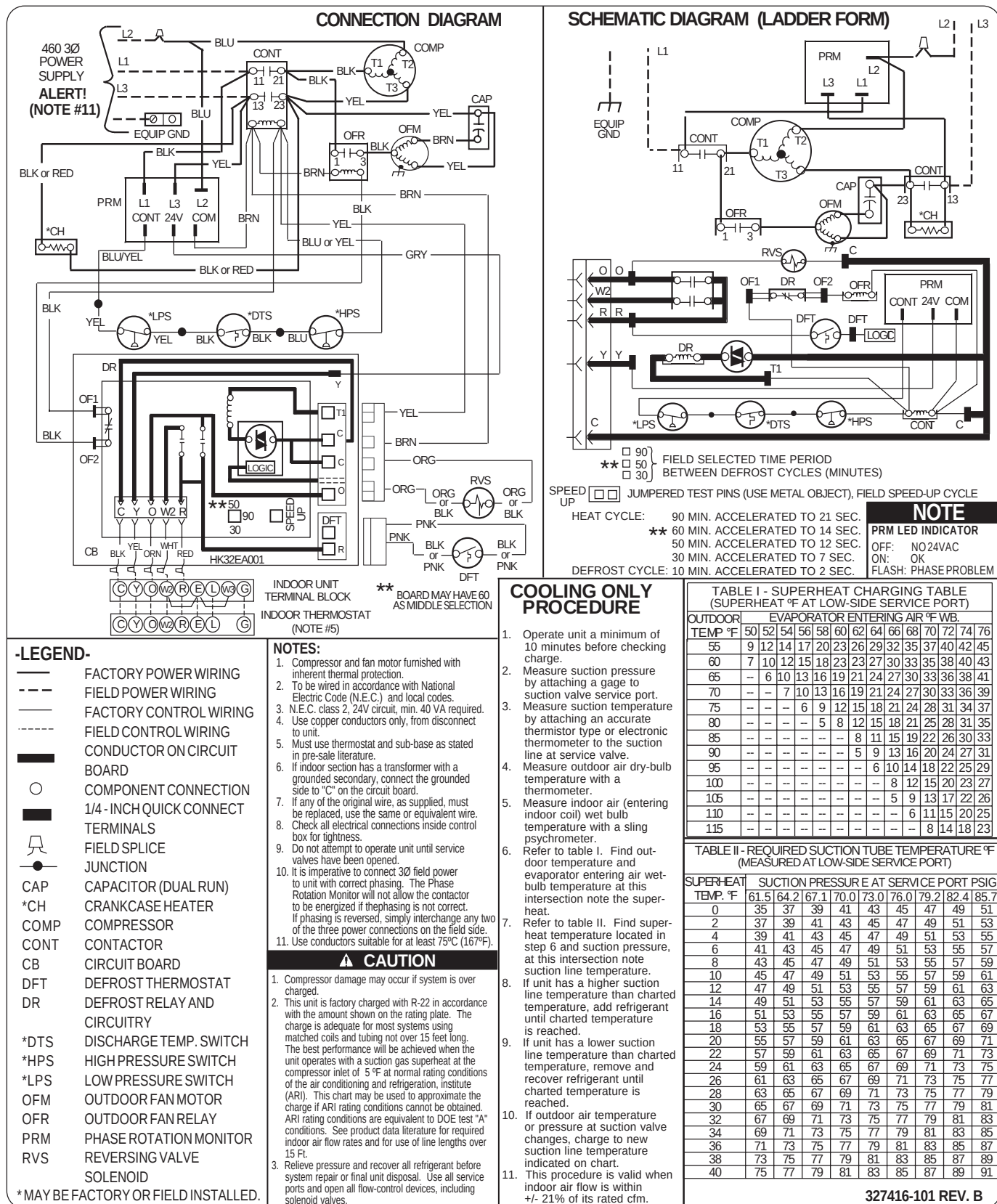
Fig. 7—Label Wiring 327416-101
