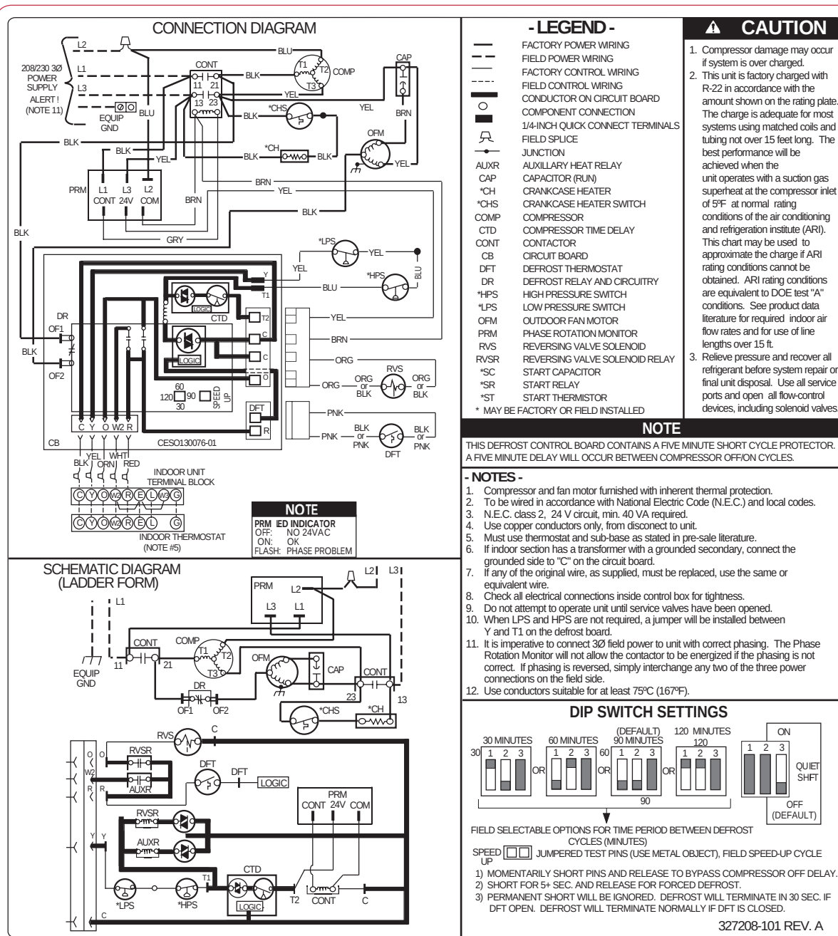
Fig. 2—Label Wiring 327208-101
