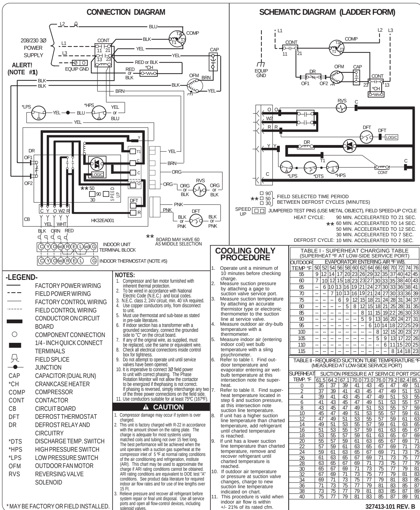
Fig. 4—Label Wiring 327413-101
