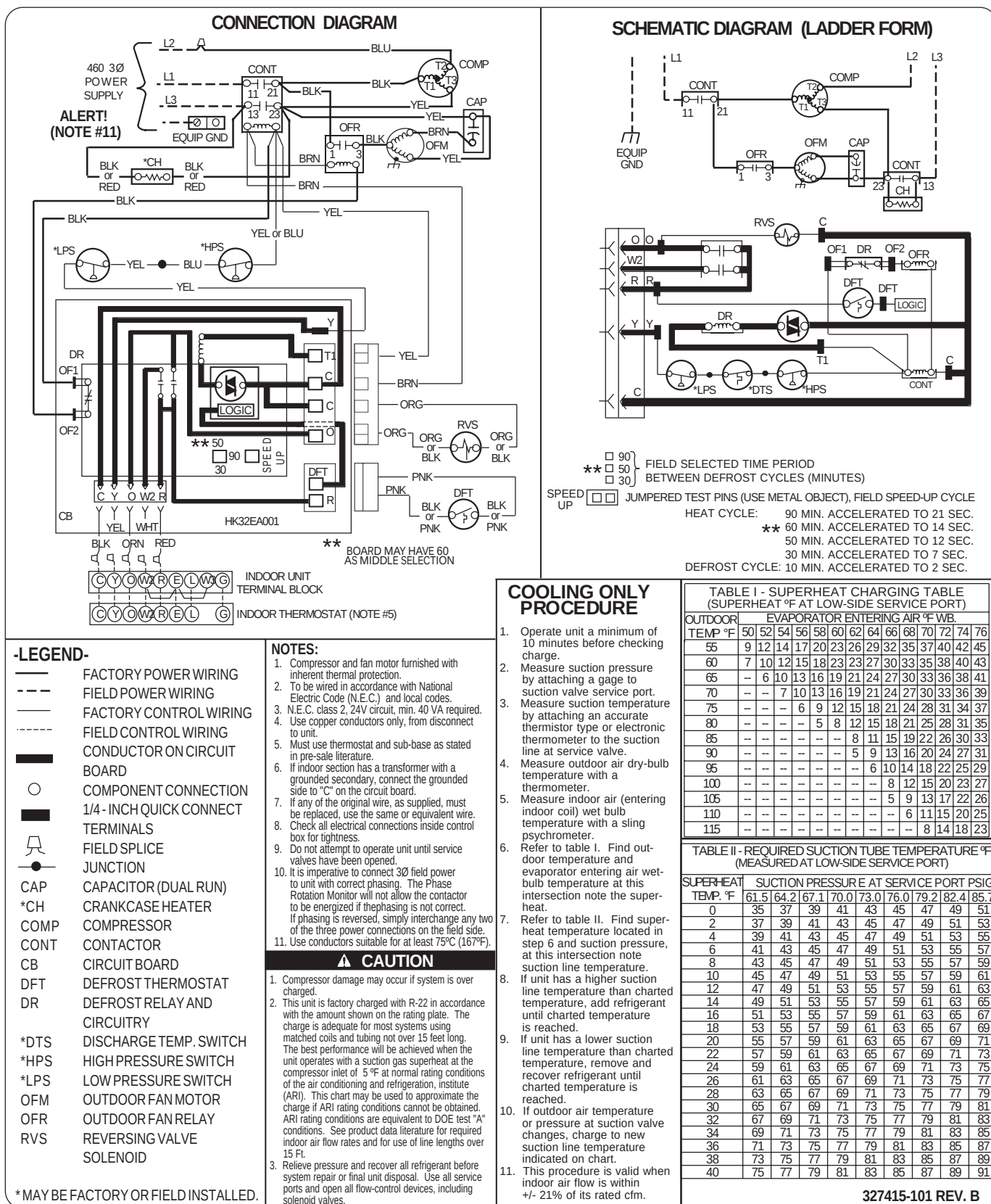
Fig. 6—Label Wiring 327415-101
