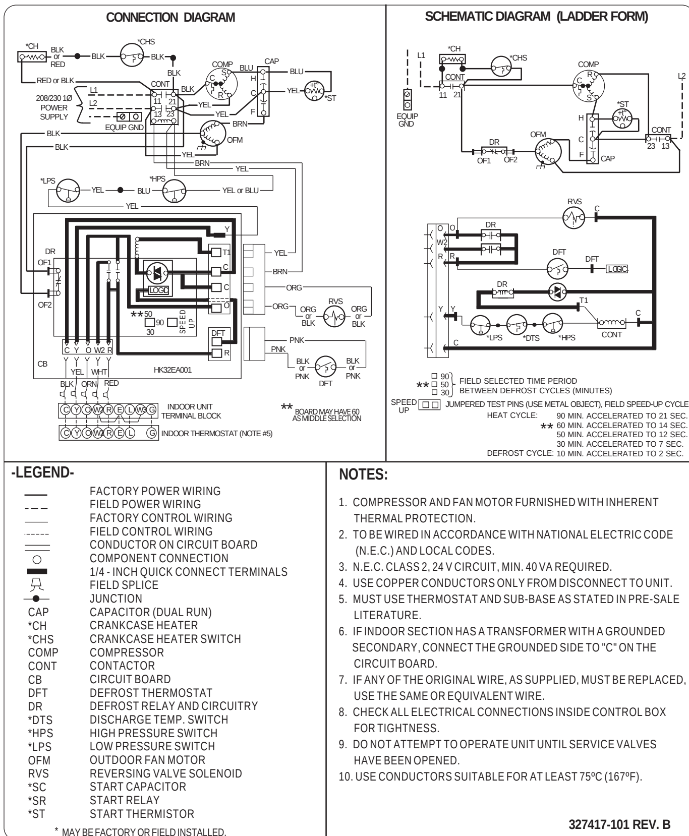
Fig. 8—Label Wiring 327417-101
