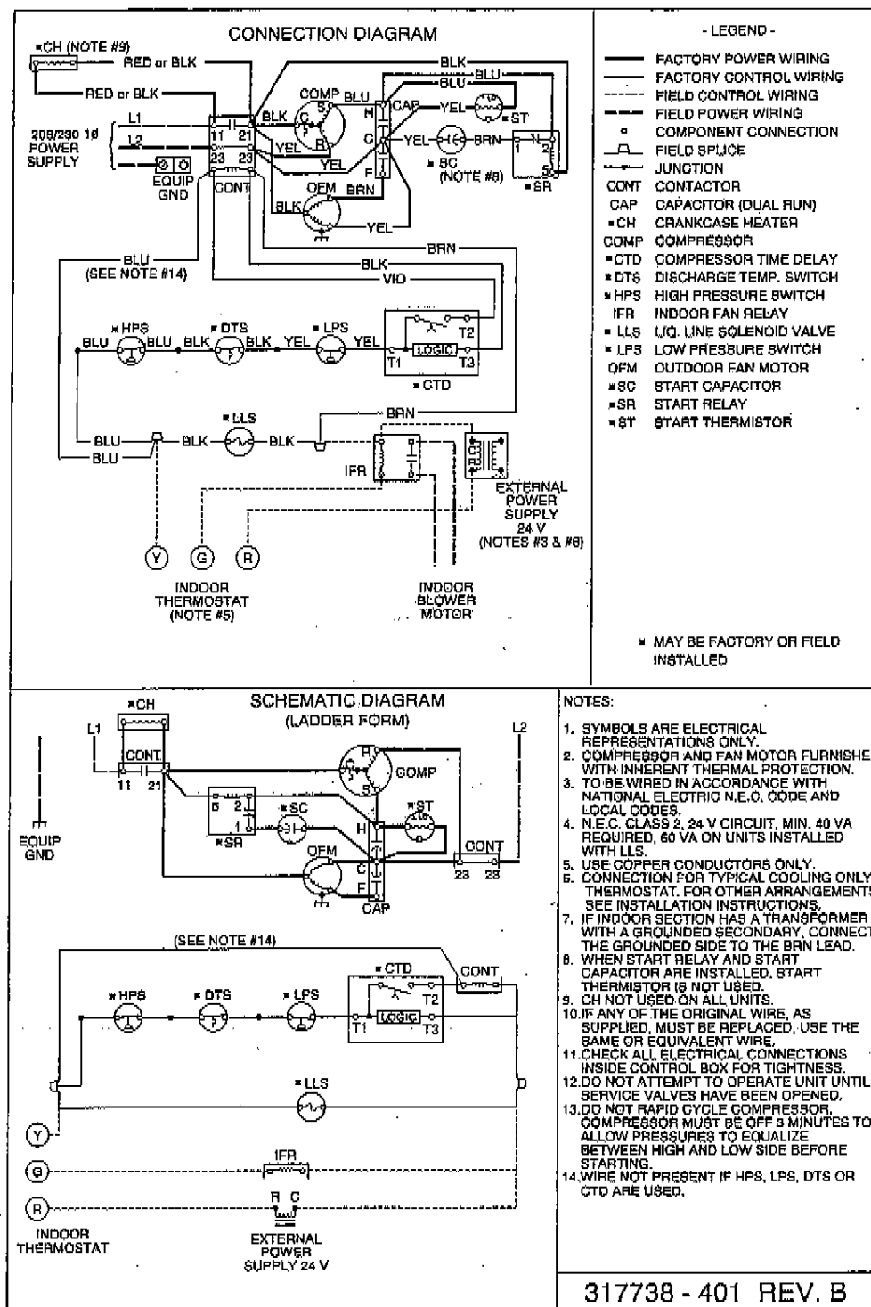
Fig. 1—38CK(M)018-048 208-230v, 1 Phase, 60 Hertz
