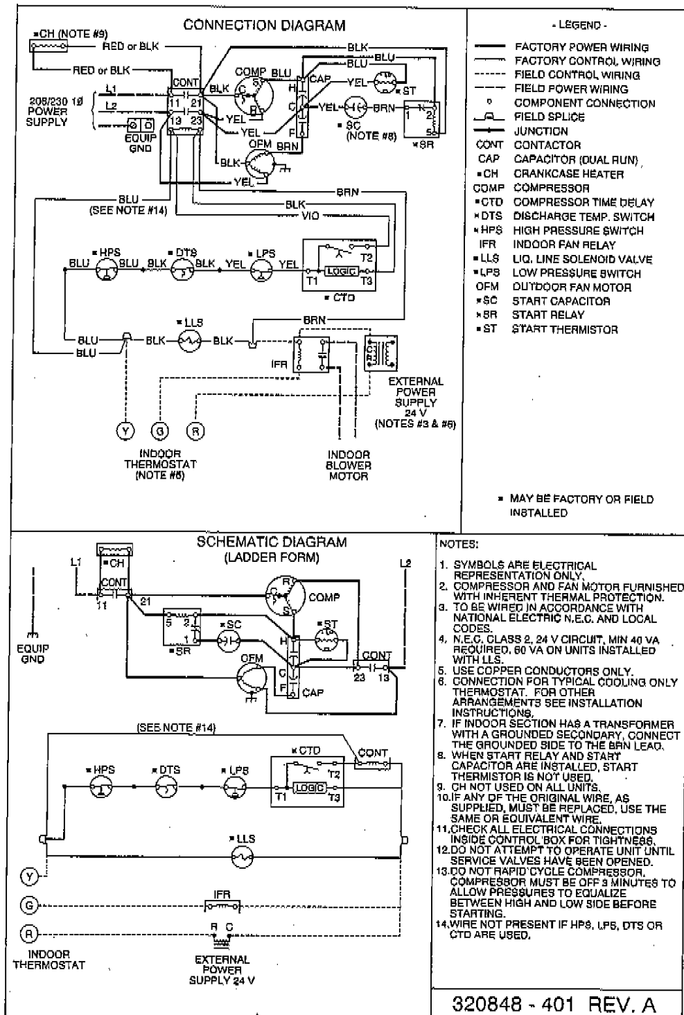
Fig. 2—38CK060 208-230v, 1 Phase, 60 Hertz
