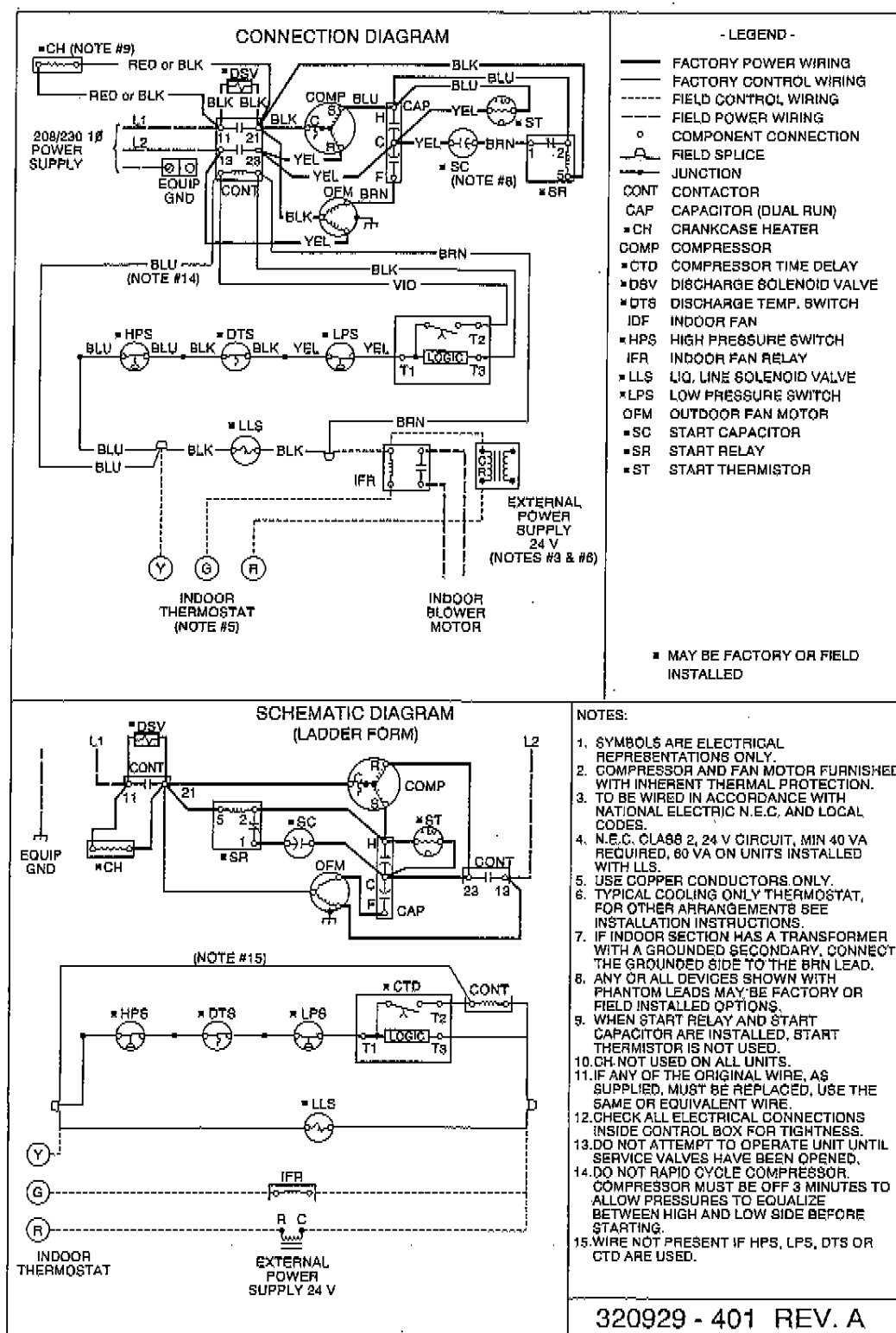
Fig. 2—38TRA060 208/230v, 1 Phase, 60 Hertz
